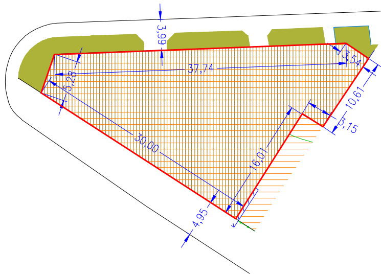
PLANTA A.A. 4-2
