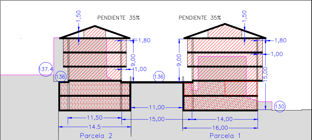
SECCION A
