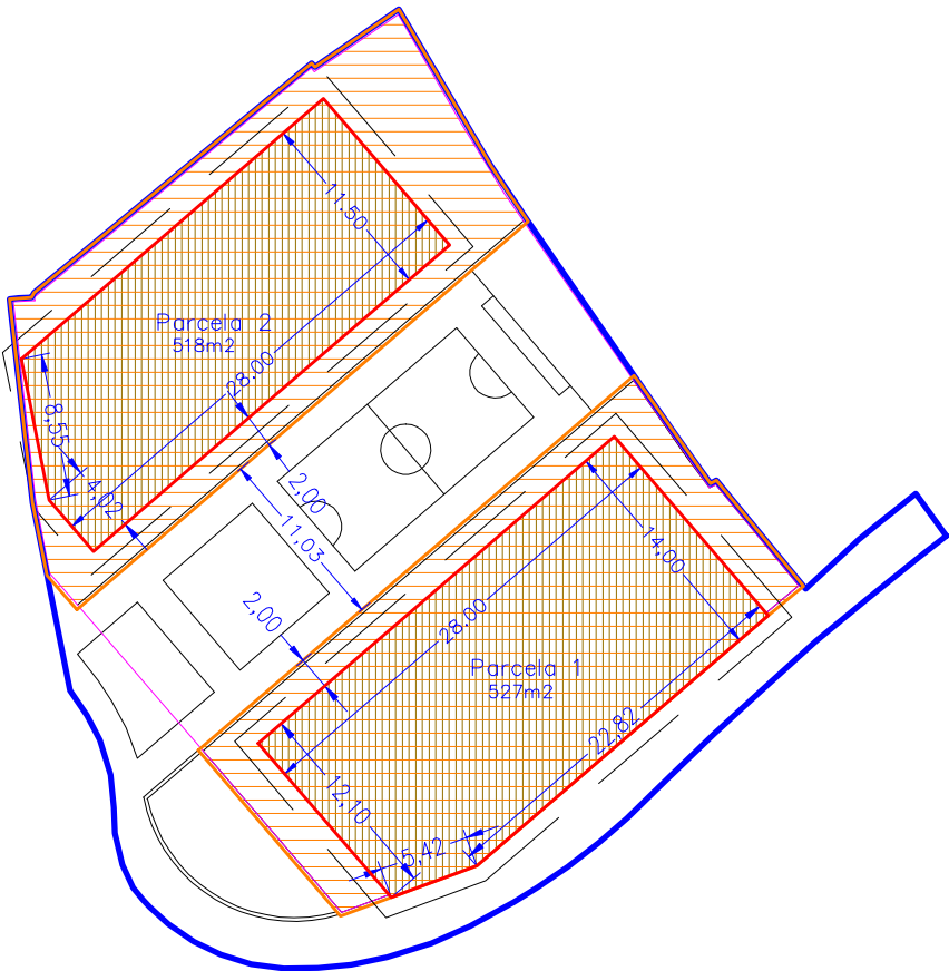
PLANTA A.A. 4-1
