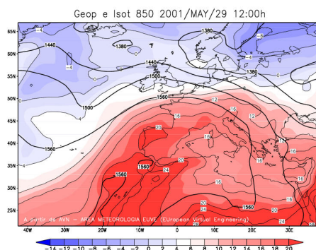
5.3, 5.4 eta 5.5 irudiak. Geopotenziala eta isotermak 850 mb-tara. Figuras 5.3, 5.4 y 5.5. Geopotencial e isotermas a 850 mb.
