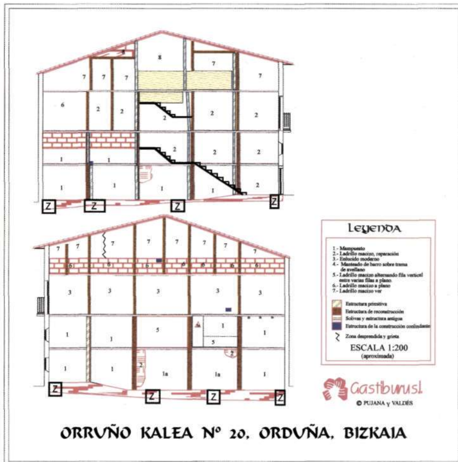
Orruño kaleko 20. zenbakiko eraikinaren barneko egitura (Orduña).
