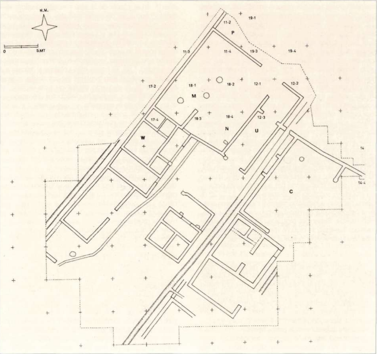
Aloriako finkamendu erromatarren Oin Nagusia. Eraikuntza egiturak.
