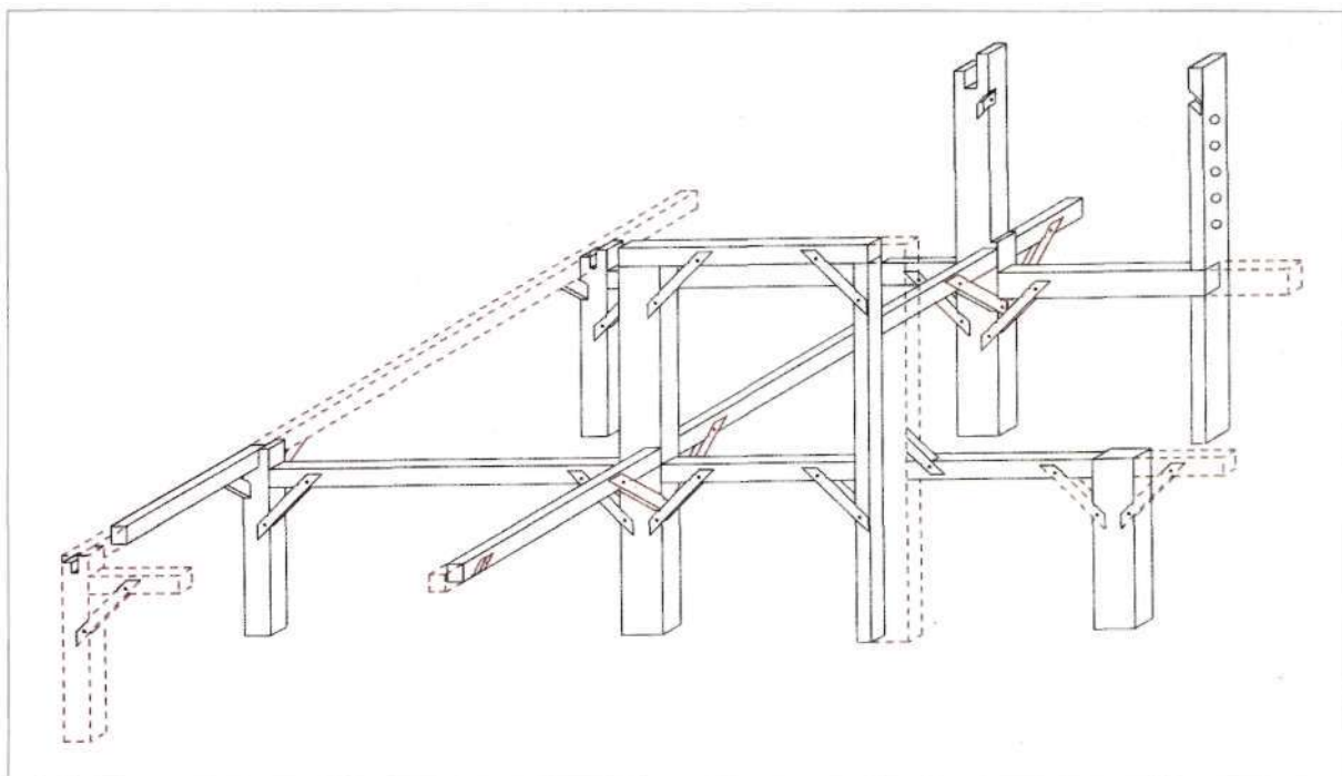
Habe-dolarearen hondakinak Etxenagusia Baserriaren barneko egituran.
