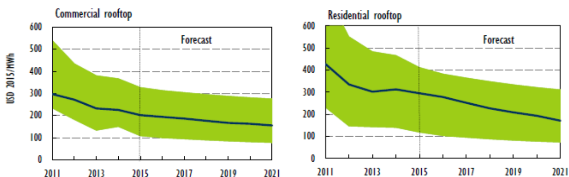
Gráfico 15. Evolución del coste de generación (LCOE) en instalaciones fotovoltaicas de tipo comercial y residencial
