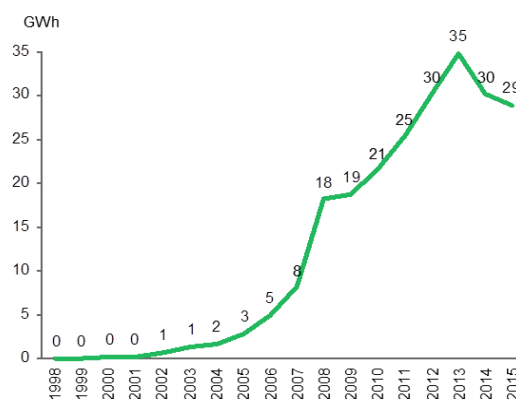
Gráfico 7. Evolución de la producción fotovoltaica eléctrica en Euskadi (GWh; 1998-2015)
