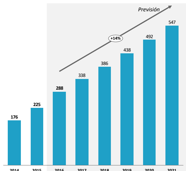
Gráfico 13. Previsiones de evolución de la capacidad de energía solar fotovoltaica (GW)
