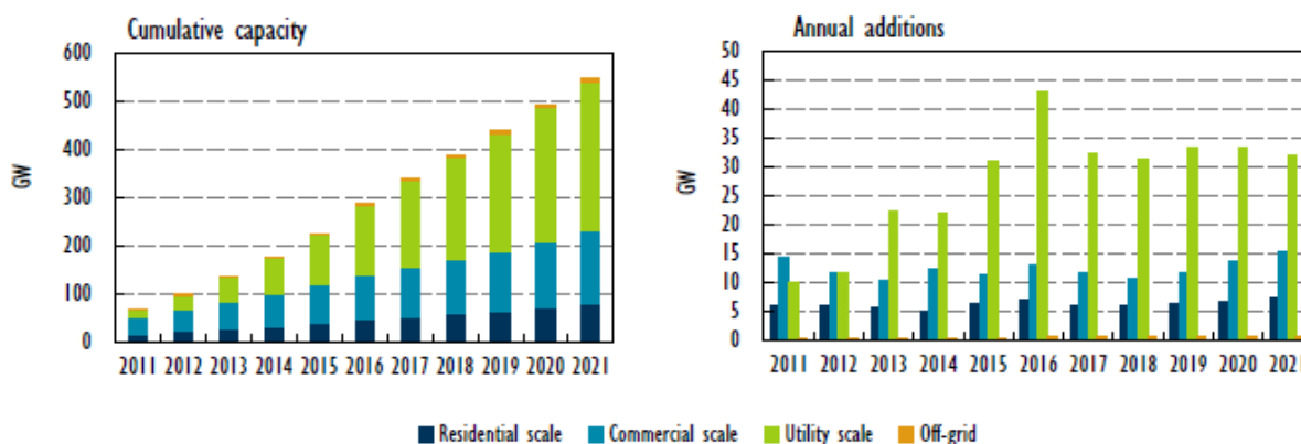
Gráfico 14. Evolución de la capacidad solar fotovoltaica instalada (acumulada y anual), por segmentos
