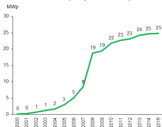
Gráfico 6. Evolución de la capacidad fotovoltaica instalada en Euskadi (MWp; 2000-2015)
