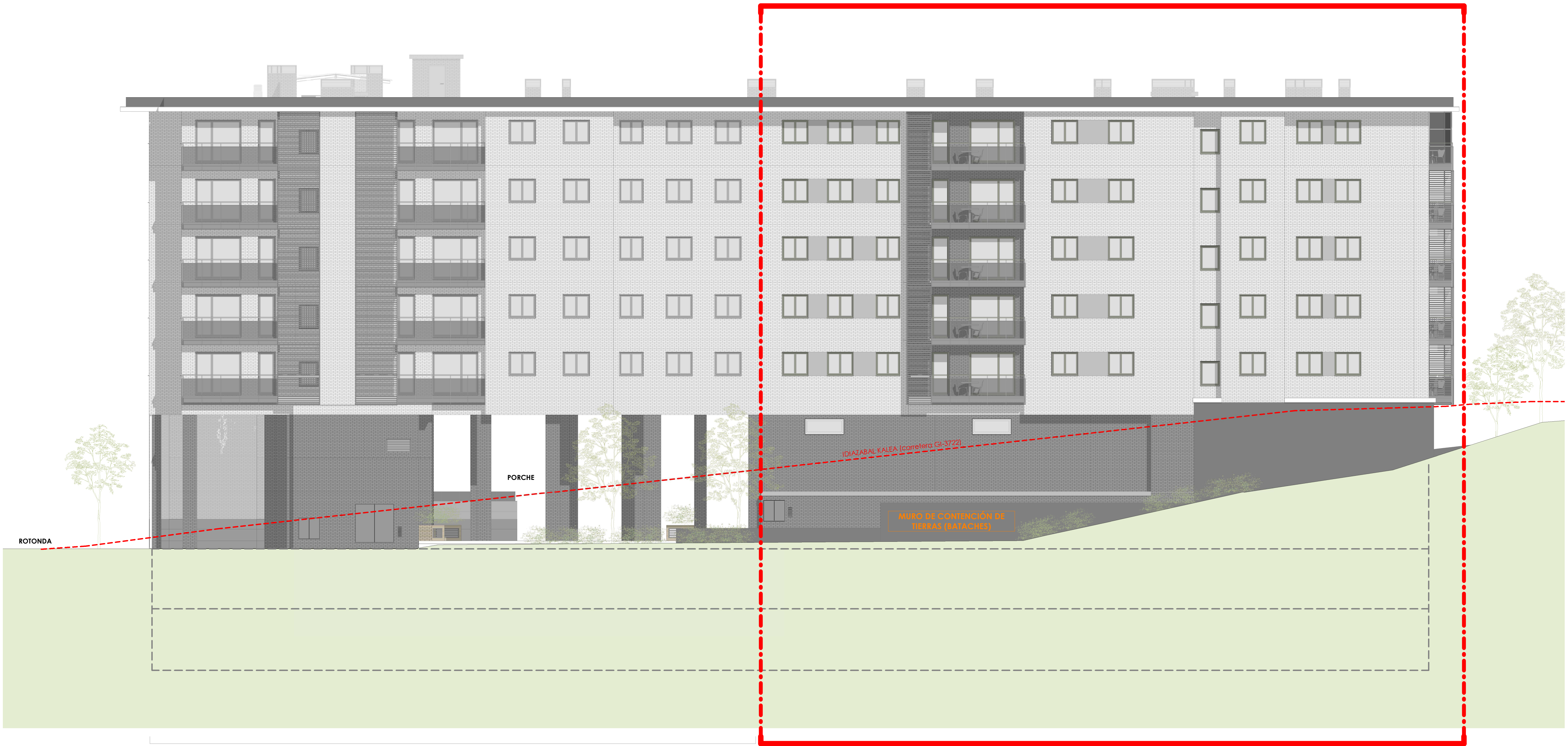
EDIFICIO VPO PARCELA UD1.2
