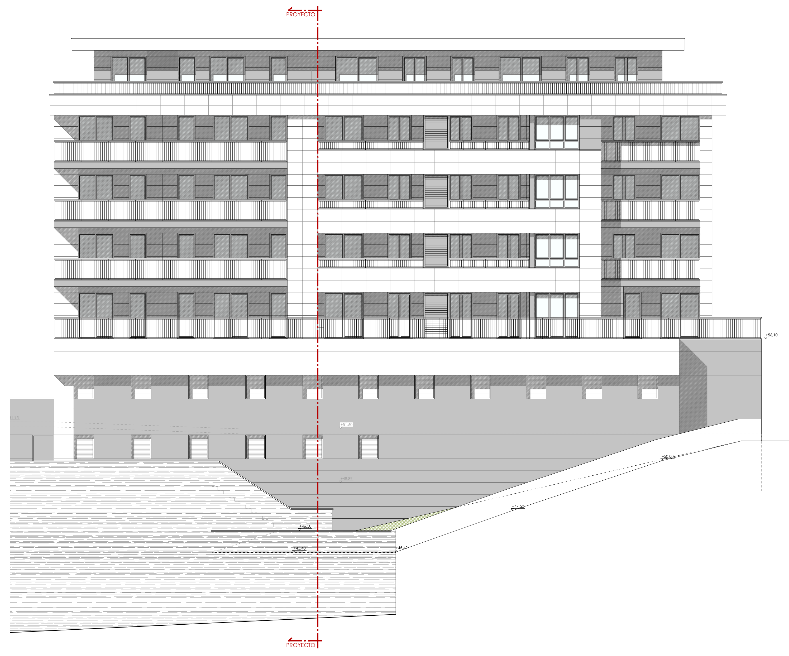
ALZADO SUROESTE
