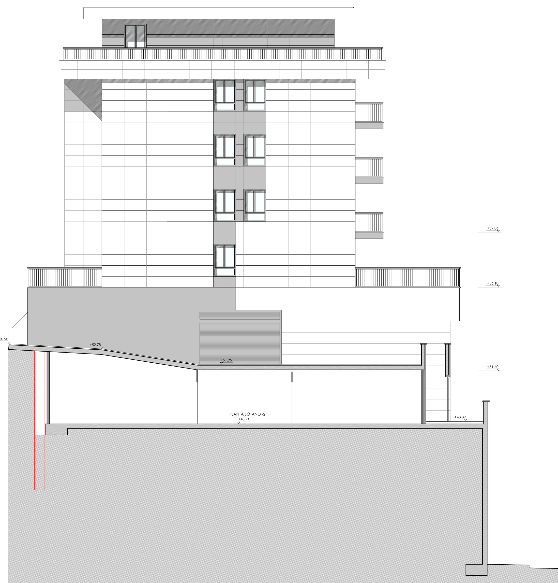
ALZADO NOROESTE
