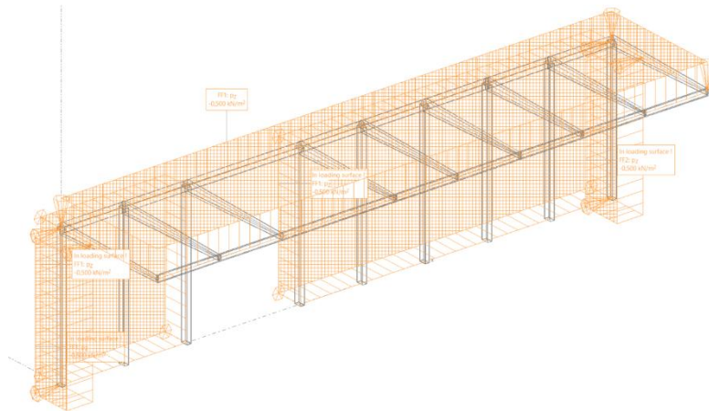
Figura 8. Definición de cargas muertas - Marquesina lateral.
