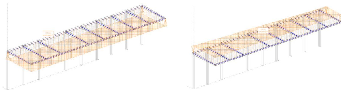
Figura 13. Cargas de viento dirección Z - Marquesina lateral.
