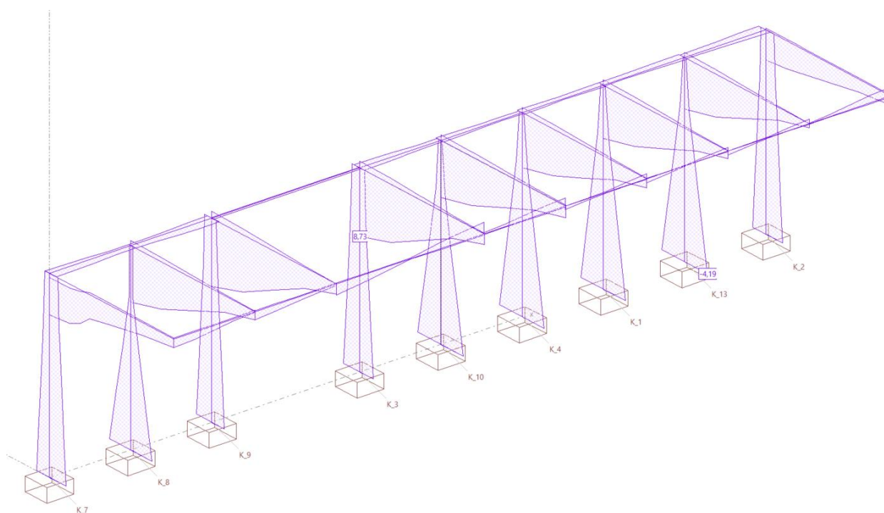
Figura 16. Envolvente ELU cortantes V_z (kN) - Marquesina lateral.
