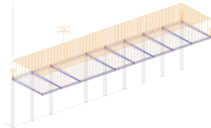
Figura 9. Sobrecargas de uso - Marquesina lateral.
