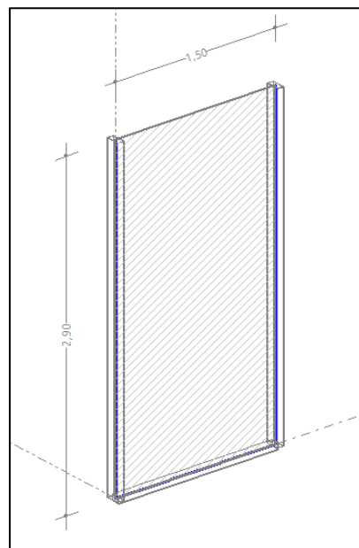
Figura 25. Dimensiones del panel OPI.
