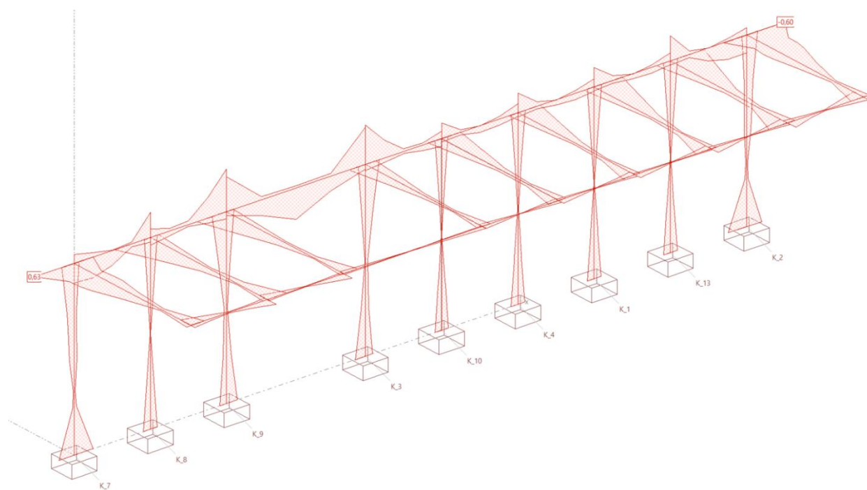
Figura 18. Envolvente ELU cortantes M_z (kNm) - Marquesina lateral.
