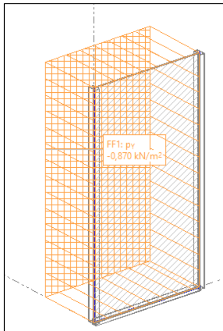
Figura 23. Cargas de viento - OPI.
