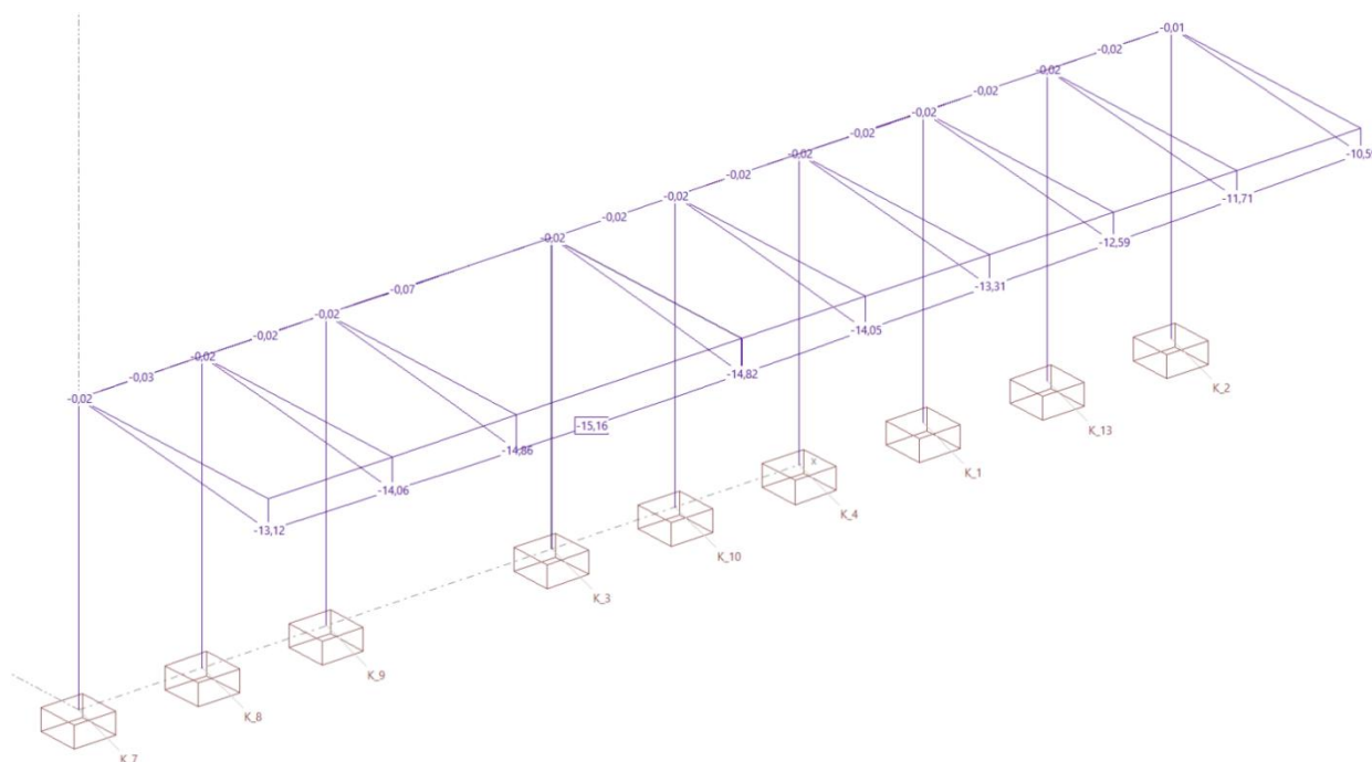
Figura 20. Deflexión de vigas - Marquesina lateral.
