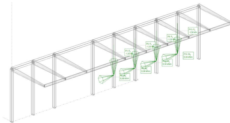
Figura 10. Sobrecargas en bancos - Marquesina lateral.
