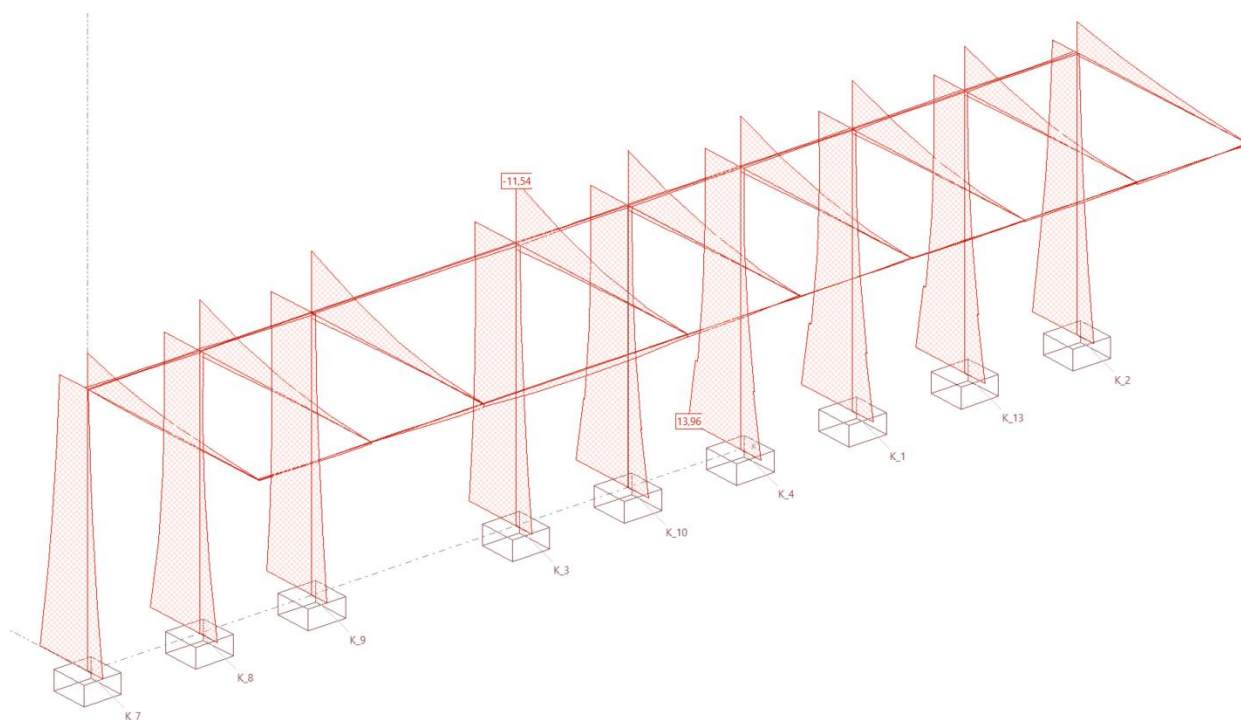
Figura 17. Envolvente ELU cortantes M_y (kNm) - Marquesina lateral.
