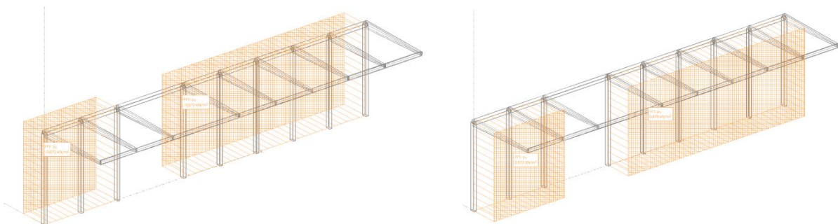
Figura 11. Cargas de viento dirección X - Marquesina lateral.
