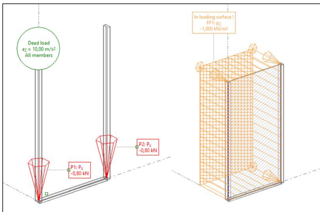
Figura 22. Peso propio y cargas muertas - OPI.
