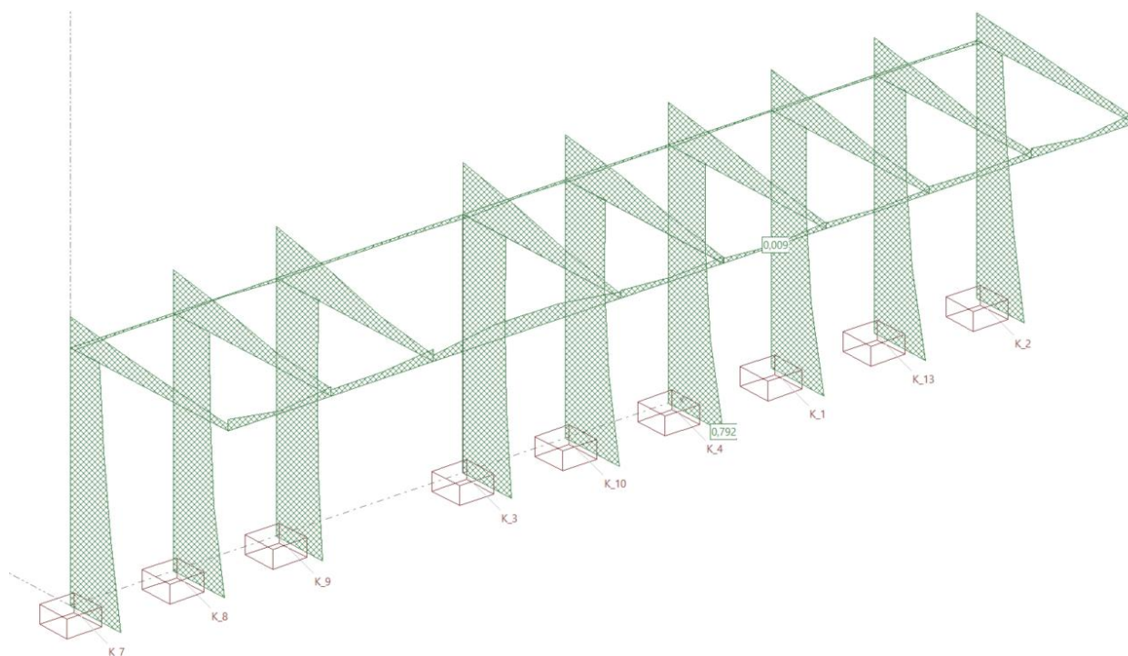
Figura 19. Eficiencia de perfiles - Marquesina lateral.
