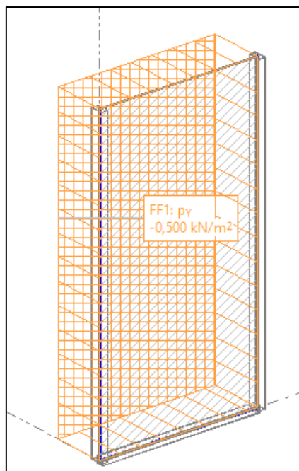
Figura 24. Cargas de uso - OPI.
