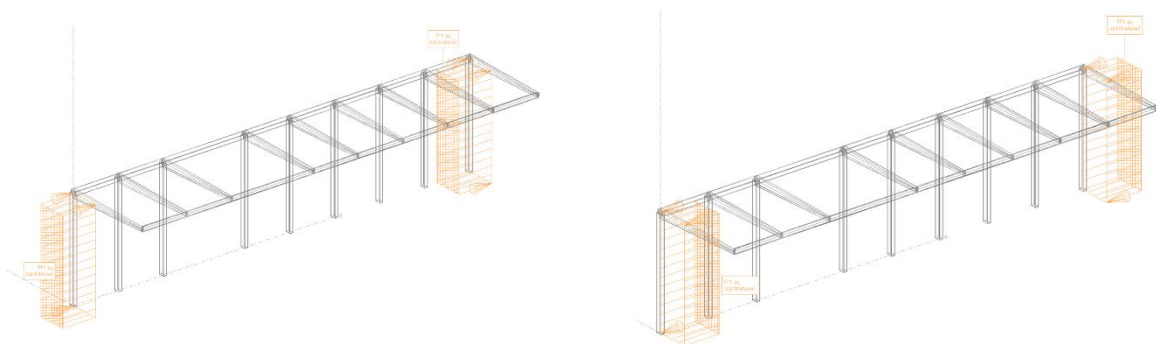
Figura 11. Cargas de viento dirección X - Marquesina lateral.
