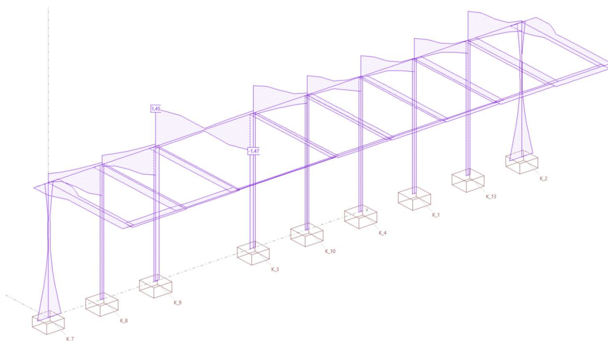
Figura 15. Envolvente ELU cortantes V_y (kN) - Marquesina lateral.
