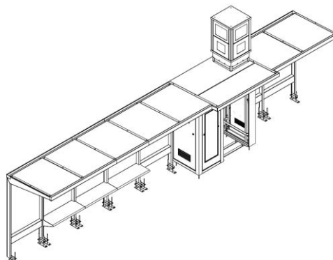
Figura 2. Ejemplo de marquesina lateral.
