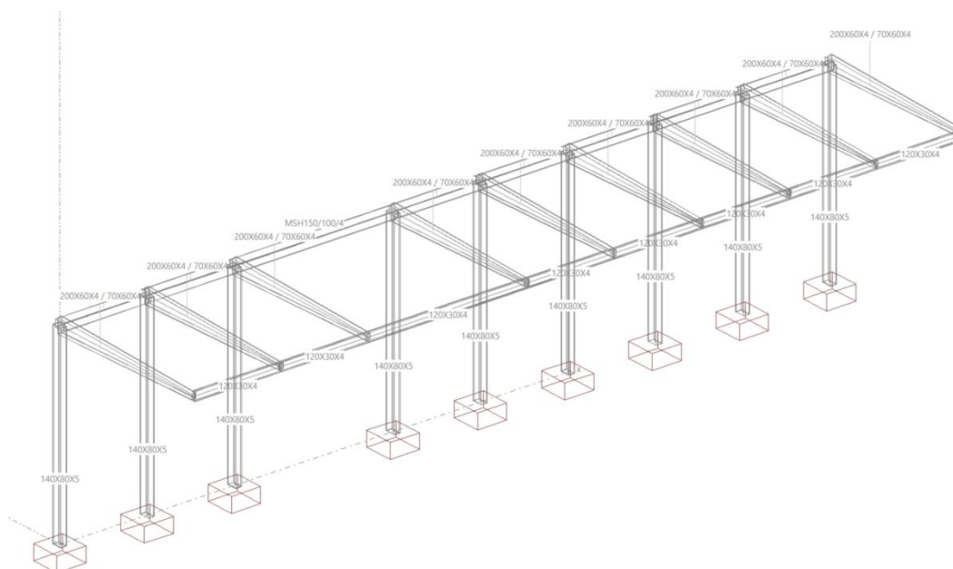
Figura 7. Definición de los perfiles metálicos - Marquesina lateral.
