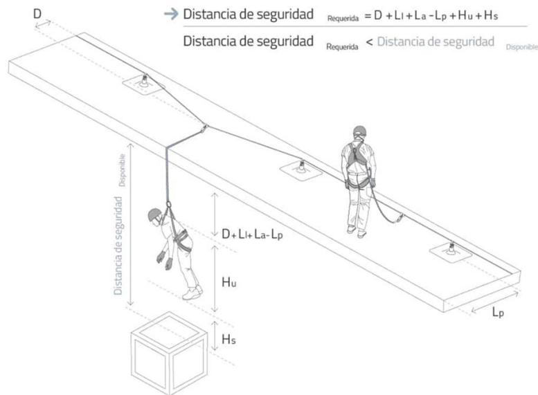
Figura 3. Distancia de seguridad para línea de vida.
