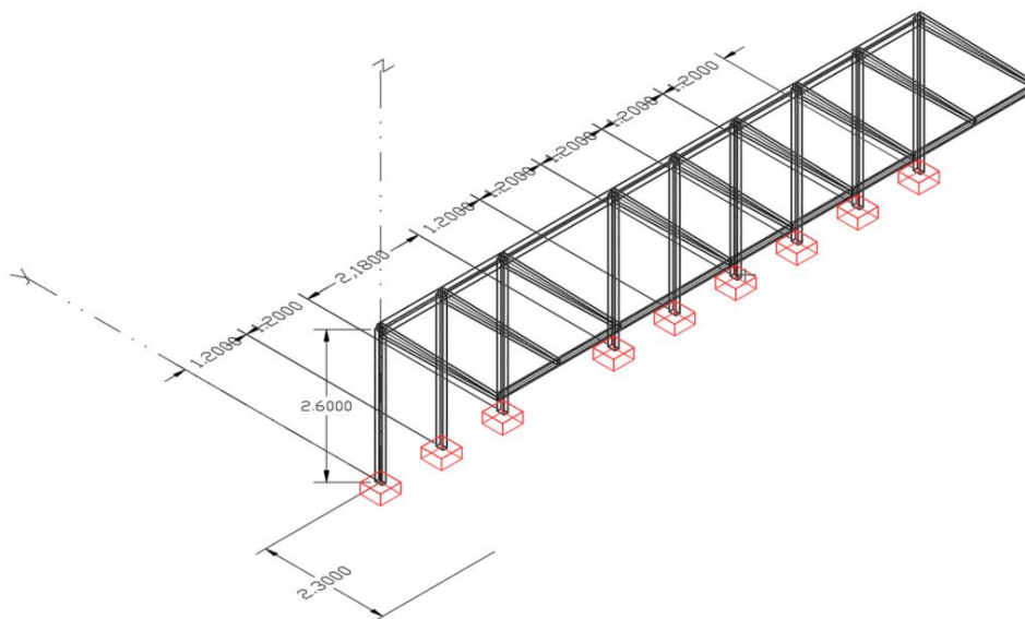
Figura 6. Modelo STATIK - Marquesina lateral.
