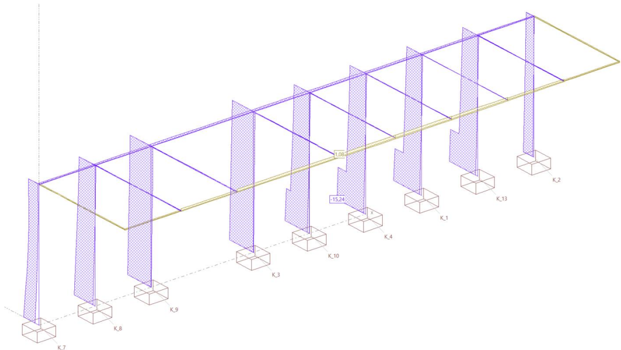
Figura 14. Envolvente ELU axiales N (kN) - Marquesina lateral.
