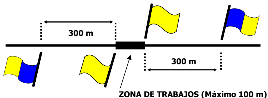
Protección en vía única de día
