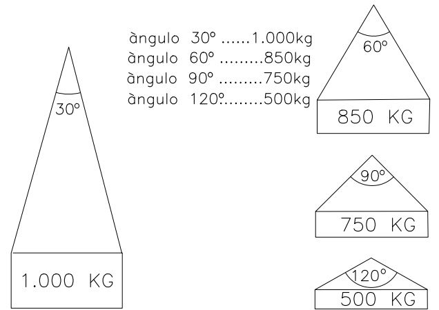
RELACION ENTRE EL ANGULO DE LA ESLINGA Y SU ACAPACIDAD DE CARGA
