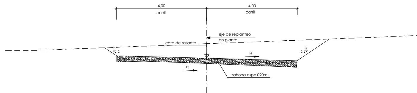
SECCIÓN TIPO DEL Pk. 0+000,000 AL 0+050,000 ESCALA 1:50
