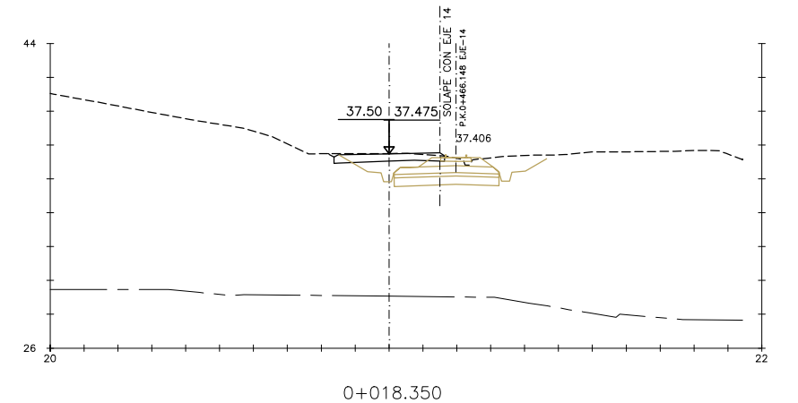
PERFILES TRANSVERSALES ESCALA 1:200
