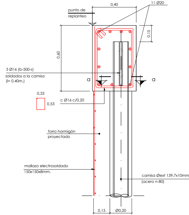
detalle 1. viga de atado en coronación escala 1/10
