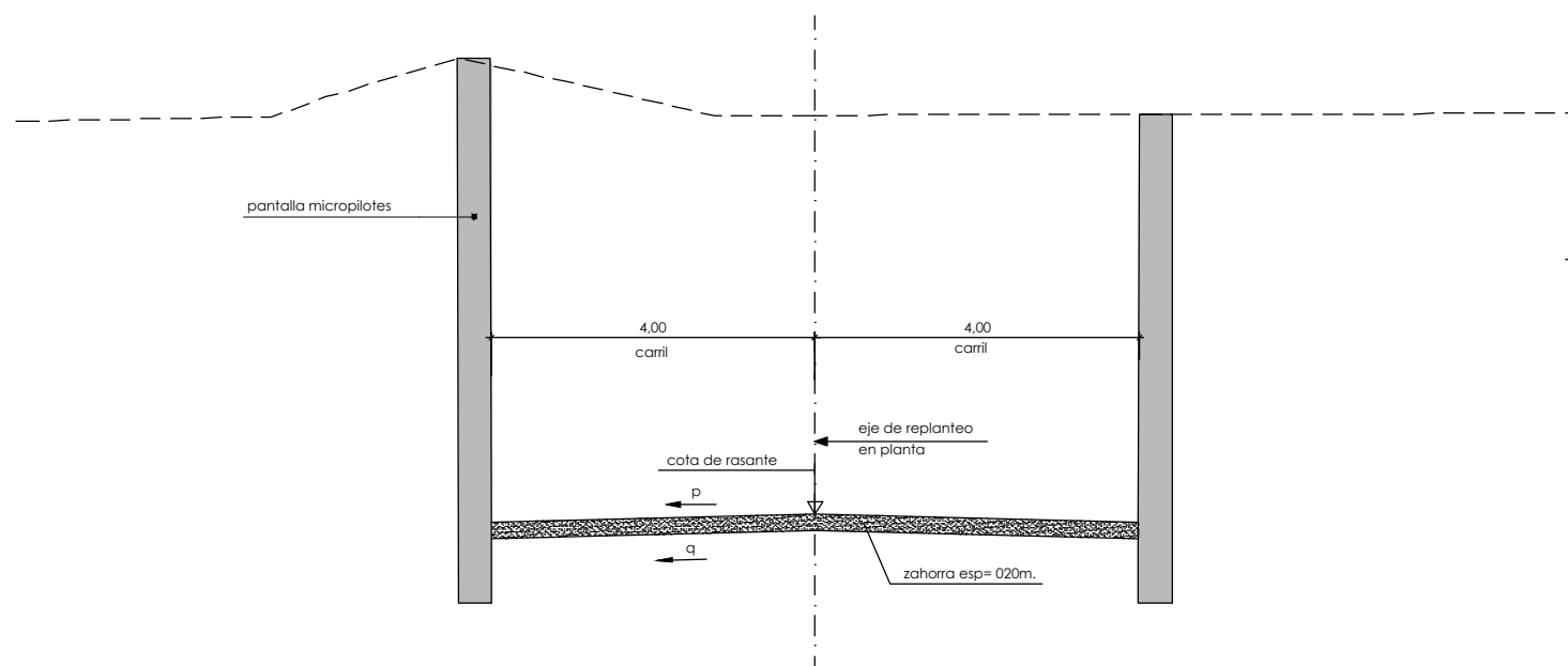
SECCIÓN TIPO DEL Pk. 0+050,000 AL 0+178,500 ESCALA 1:50
