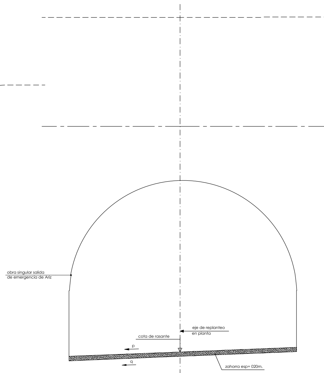
SECCIÓN TIPO DEL Pk. 0+175,000 AL 0+255,835 ESCALA 1:50
