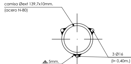
sección a-a escala 1/5
