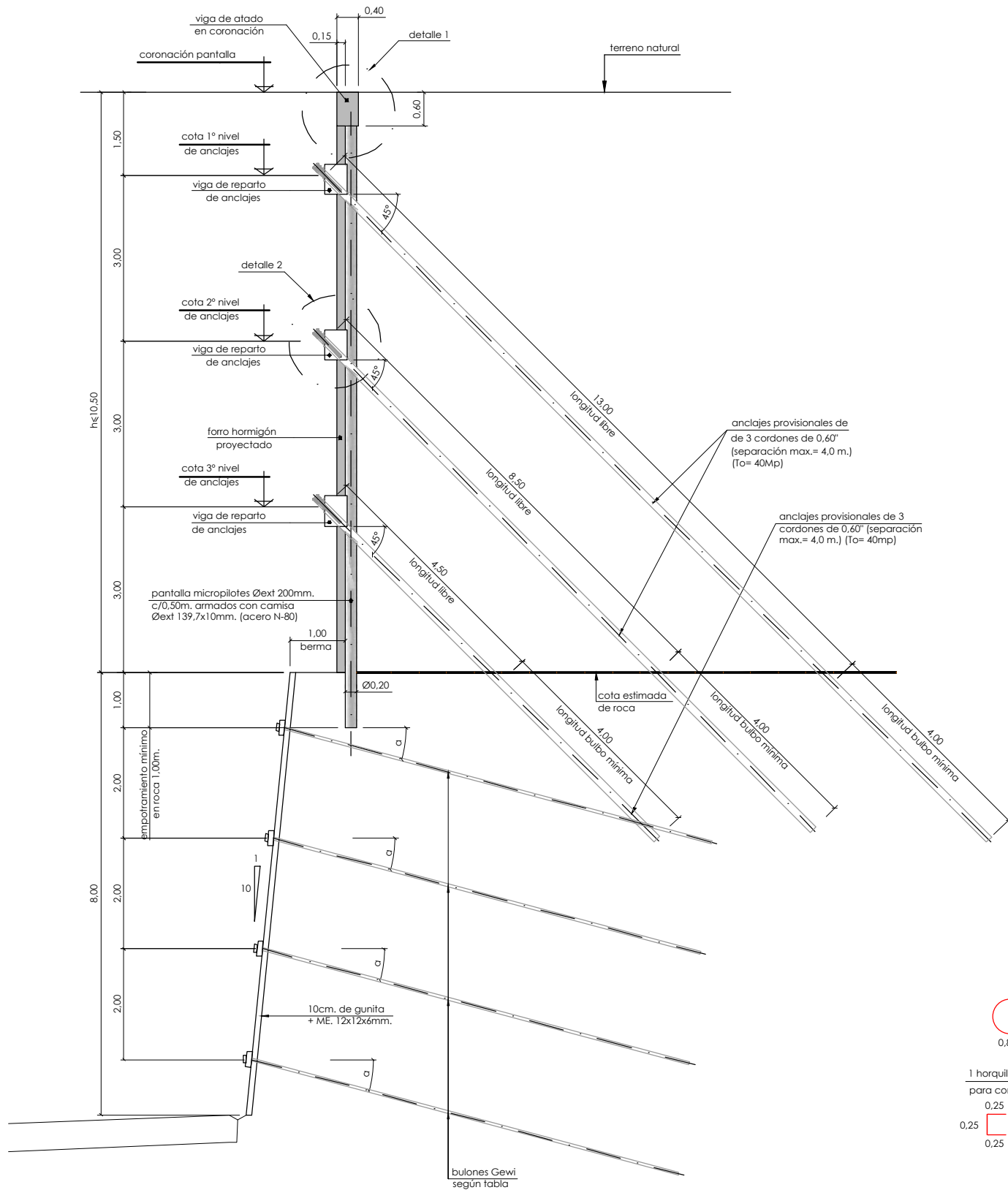
sección tipo pantalla provisional anclada escala 1/50
