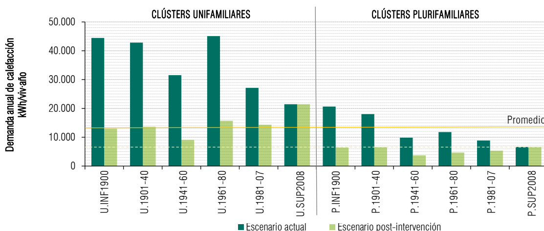
Figura 3. Demanda energética de calefacción por vivienda según clúster y escenario
