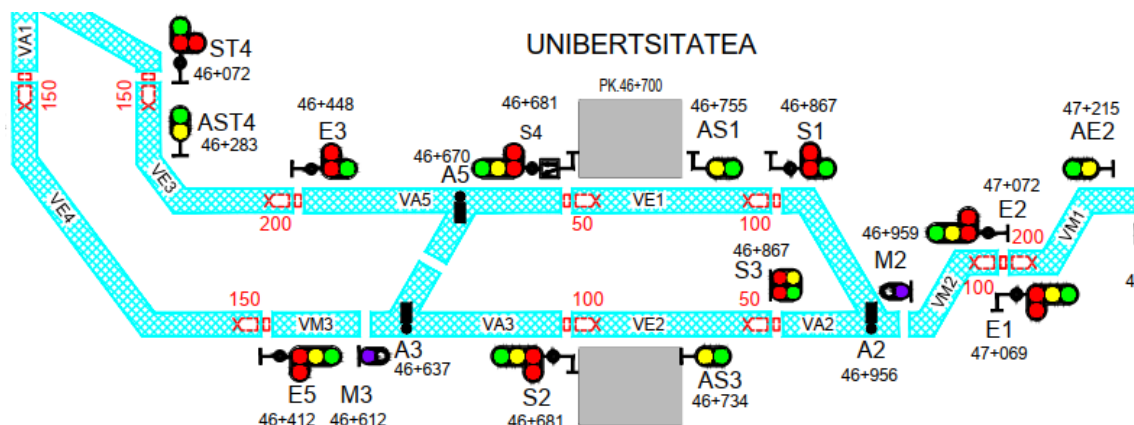
Instalaciones de seguridad en el entorno de la estación, con sus respectivos puntos kilométricos.
