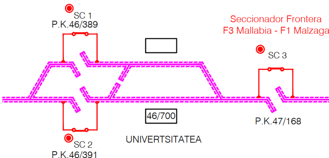
Instalaciones de electrificación en el entorno de la estación, con sus respectivos puntos kilométricos.
