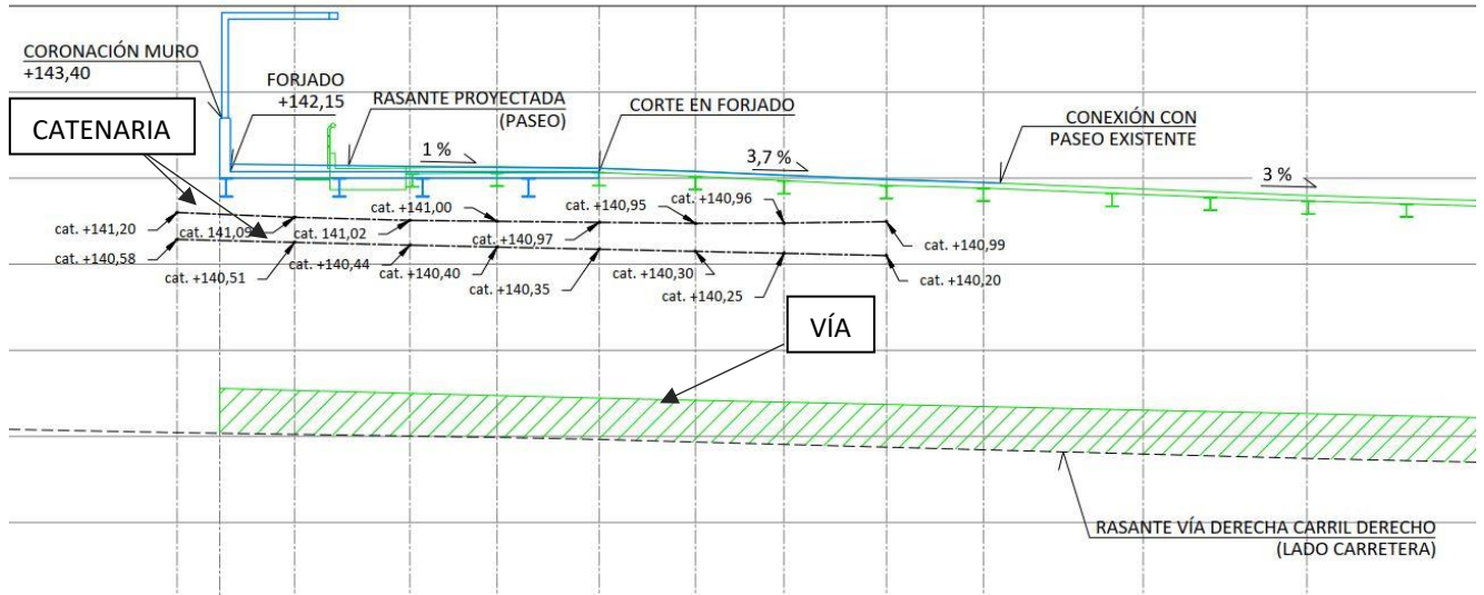
Perfil longitudinal del andén. En color gris, la vía y la catenaria de electrificación.
