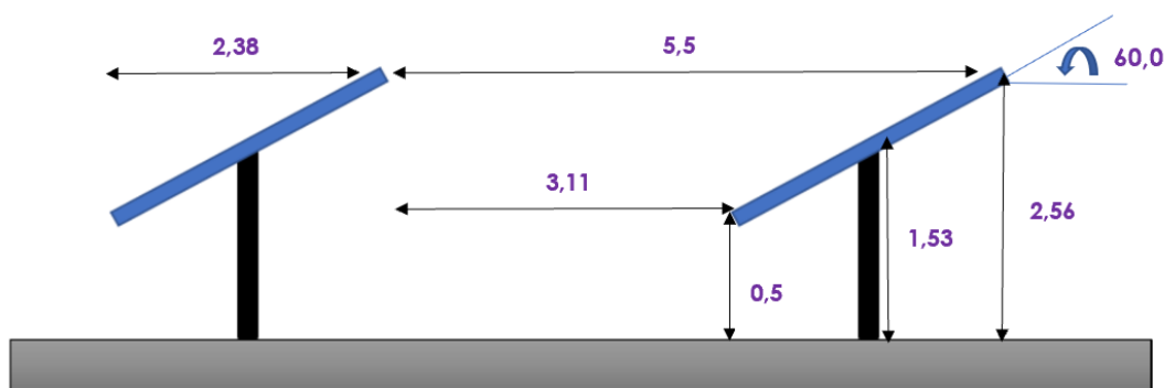
Figura 1. Diseño de estructura
