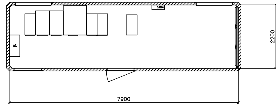
SECCIÓN B-B
