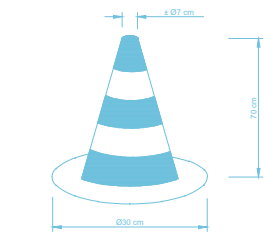
CONO BALIZAMIENTO
