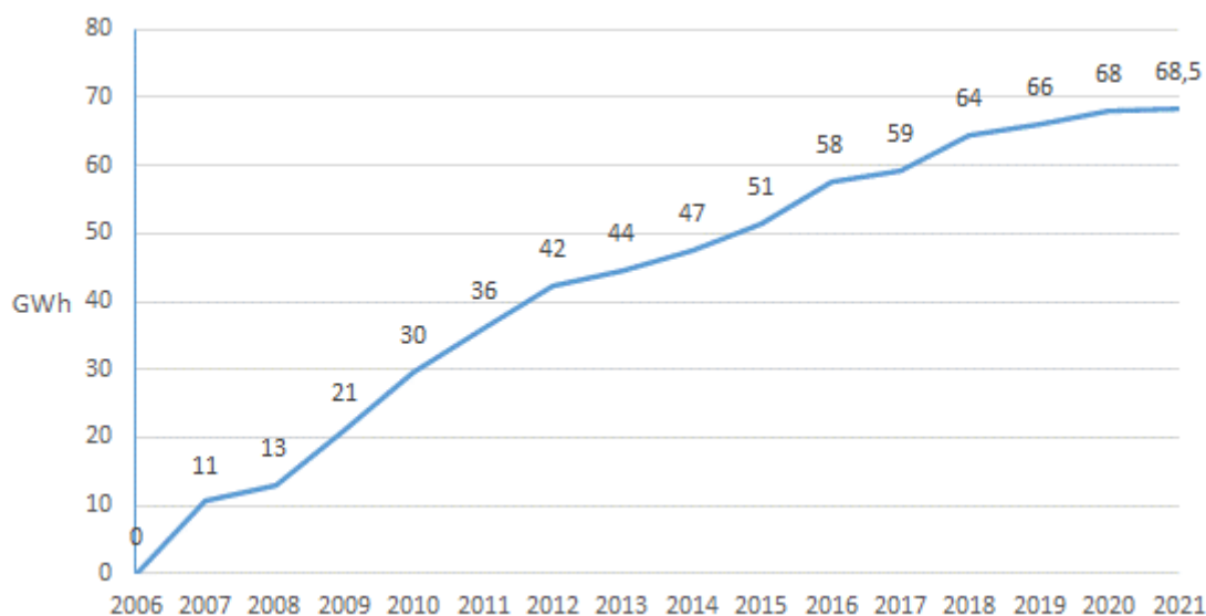
Gráfica 21. Evolución de la producción con solar térmica en Euskadi (GWh; 2005-2021)
