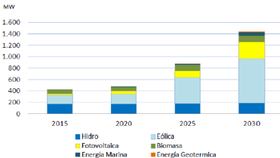
Gráfica 23. Escenario de potencia eléctrica renovable instalada en Euskadi.
