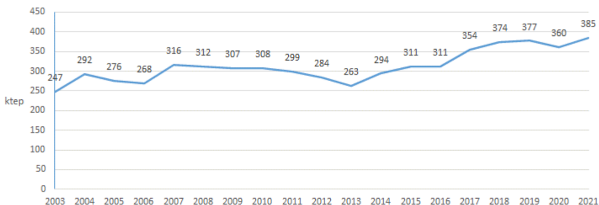
Gráfica 14. Evolución del aprovechamiento energético de la biomasa en Euskadi (GWh 2003-2021)
