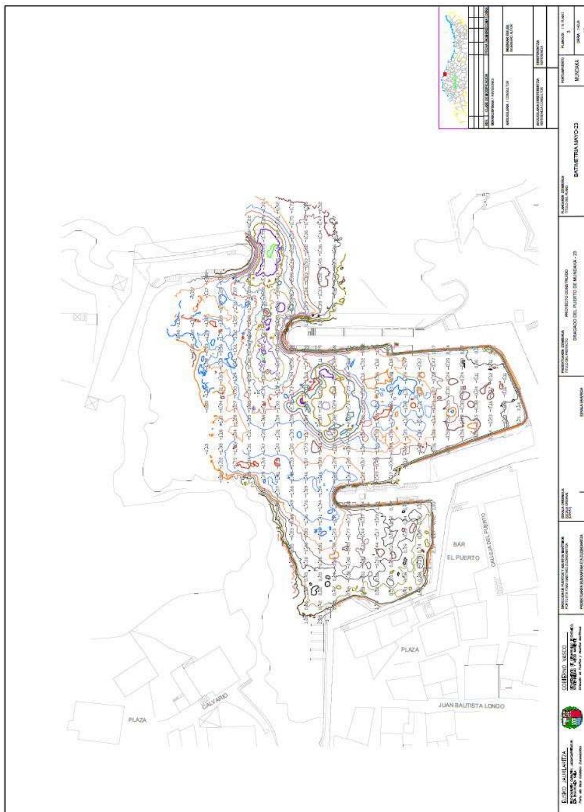
Batimetria del puerto de Mundaka
