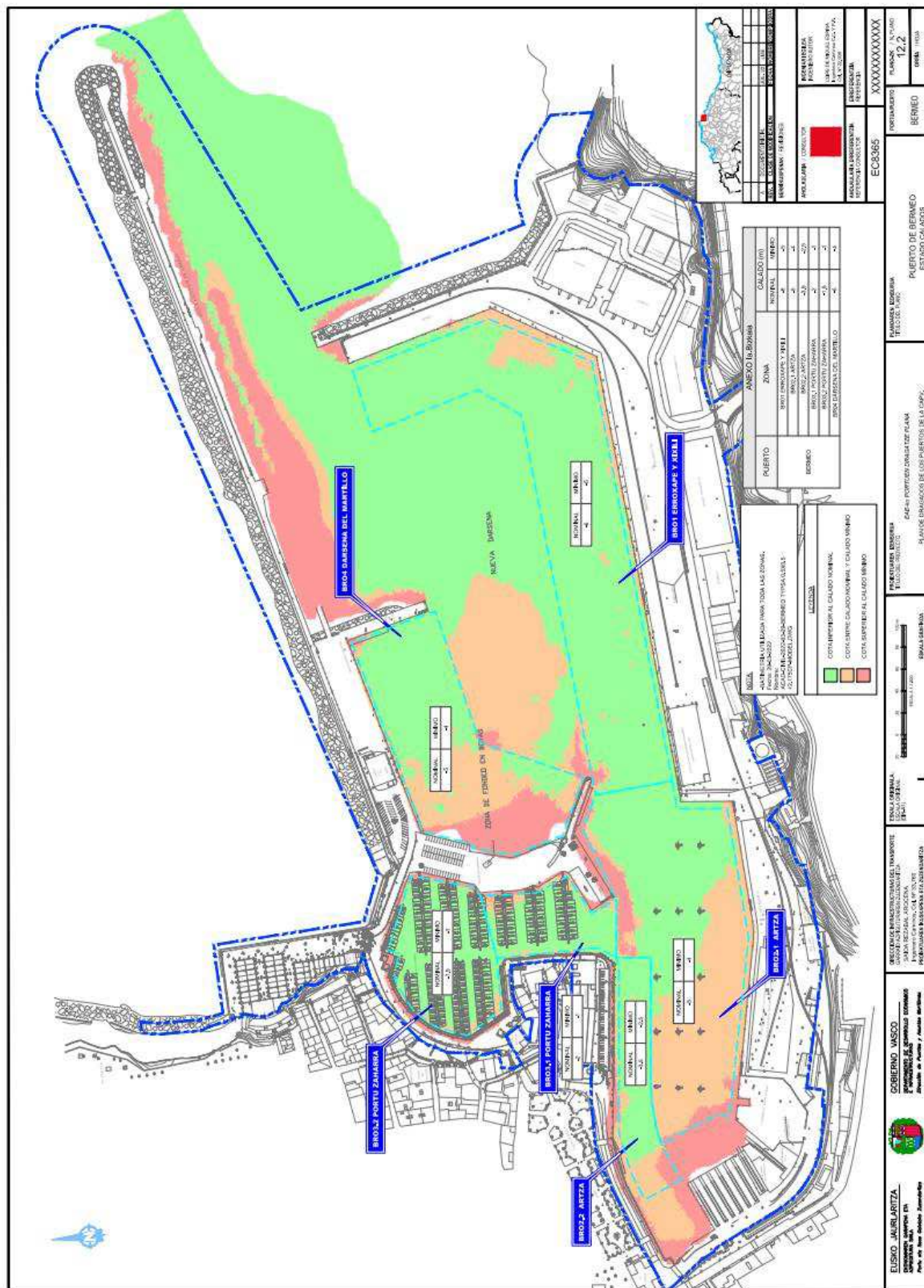
Batimetría del puerto de Bermeo.
