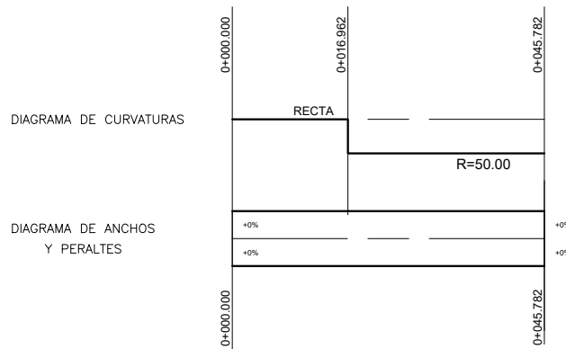
Vial 1 Fase III (Eje 107)
