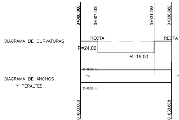
Ampliación rotonda Fase V (Eje 123)
