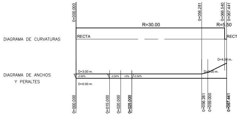
Desvío policía Fase III (Eje 105)
