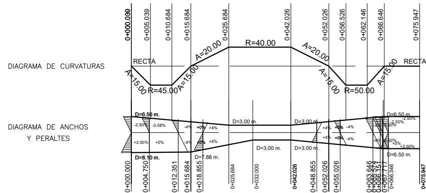
Desvío vial Fase V (Eje 158)
