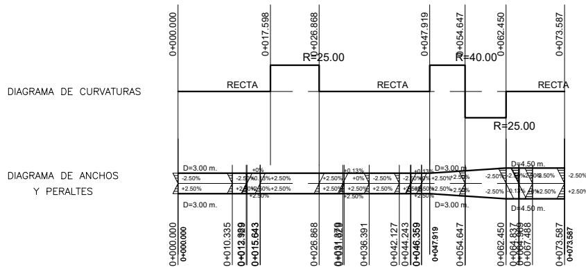
Desvío colegio Fase V (Eje 122)
