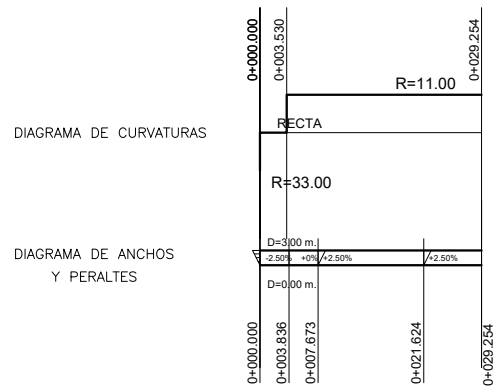
Auxiliar desvío policía Fase III (Eje 106)
