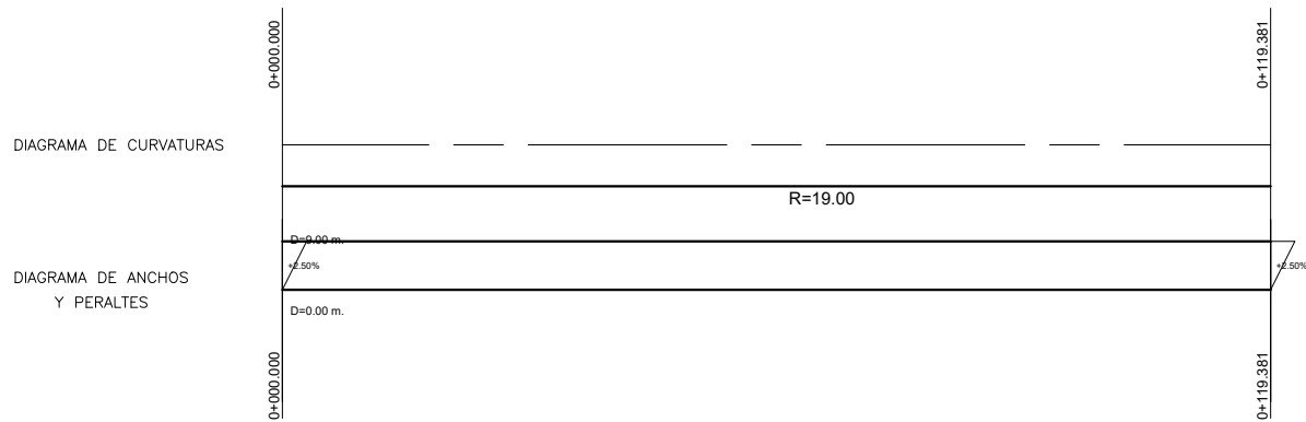
Rotonda provisional Fase III (Eje 104)
