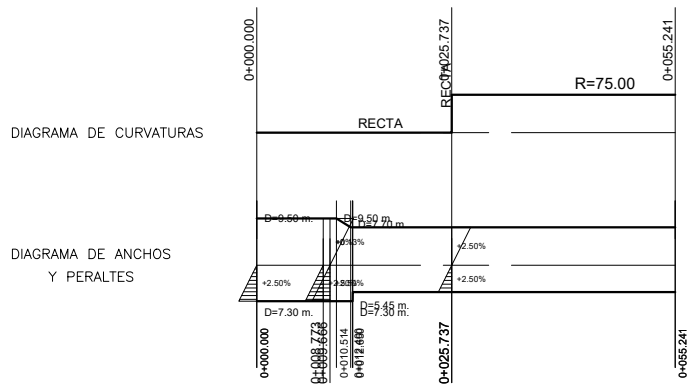
Vial 3 Fase III (Eje 109)
