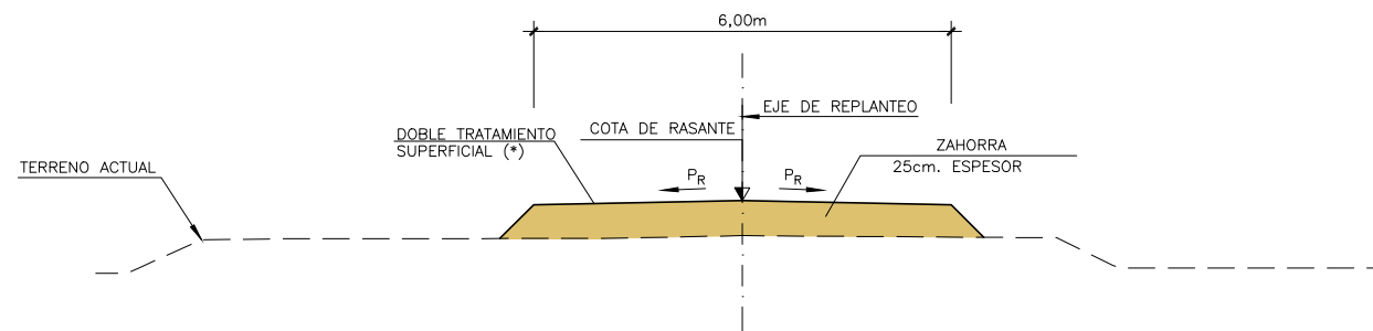
SECCIÓN TIPO CAMINOS DE ACCESO A OBRA
