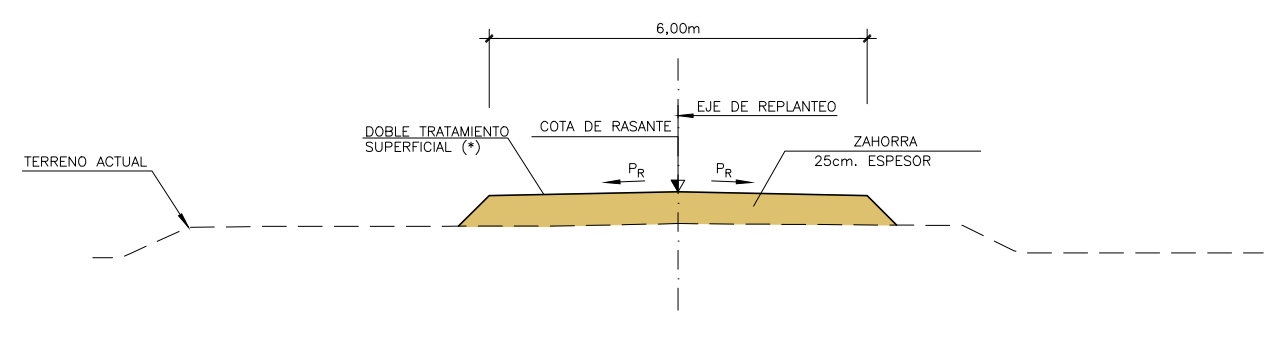
SECCIÓN TIPO CAMINOS DE ACCESO A OBRA
