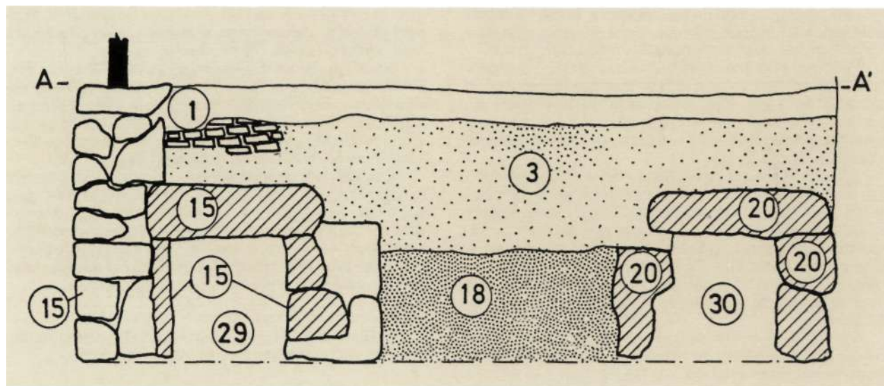
Bidebarrieta, 8. Sección A-A': Canalizaciones, siglo XIX.
