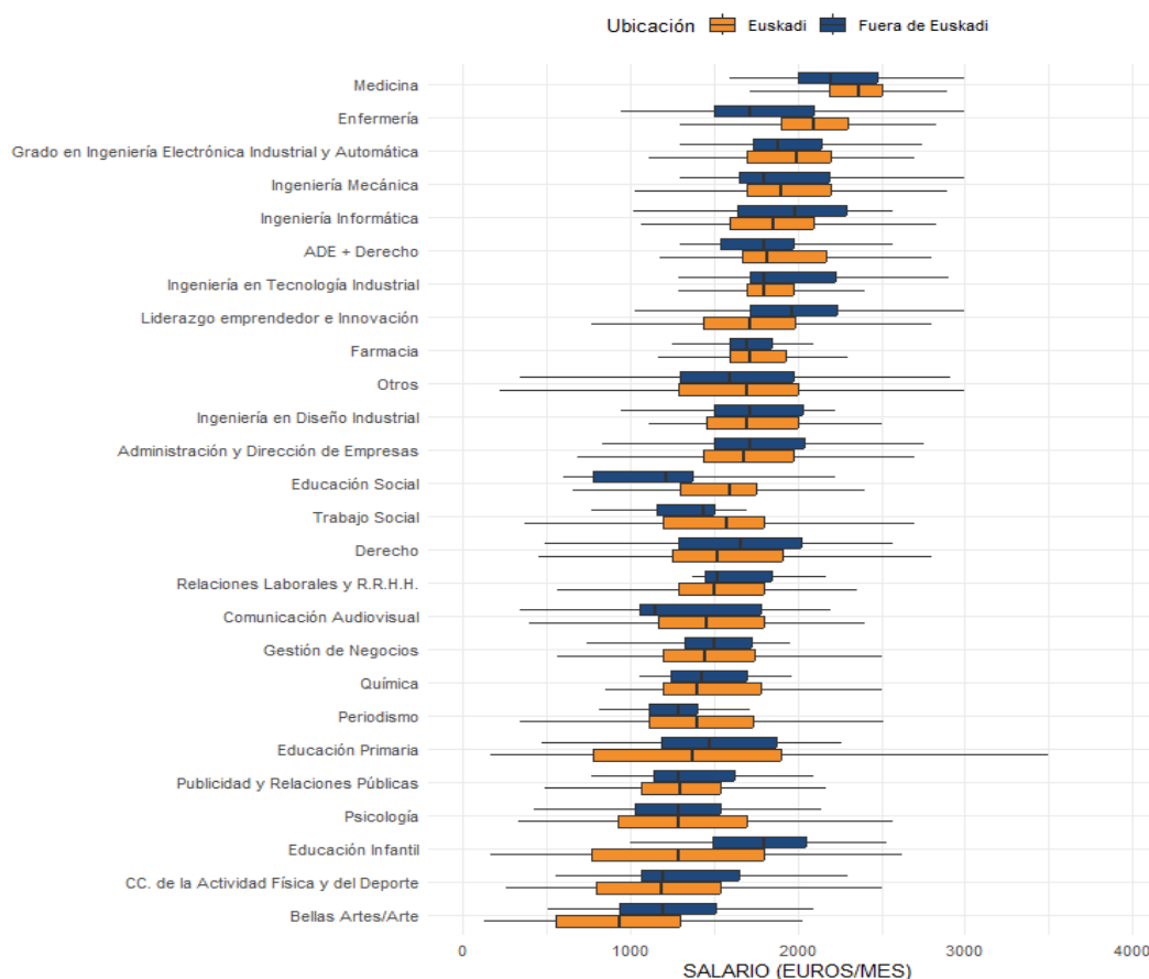
Gráfico 23. Diagrama de cajas 7 de los salarios por títulos y destino de trabajo puestos a jornada completa (euros/mes)
