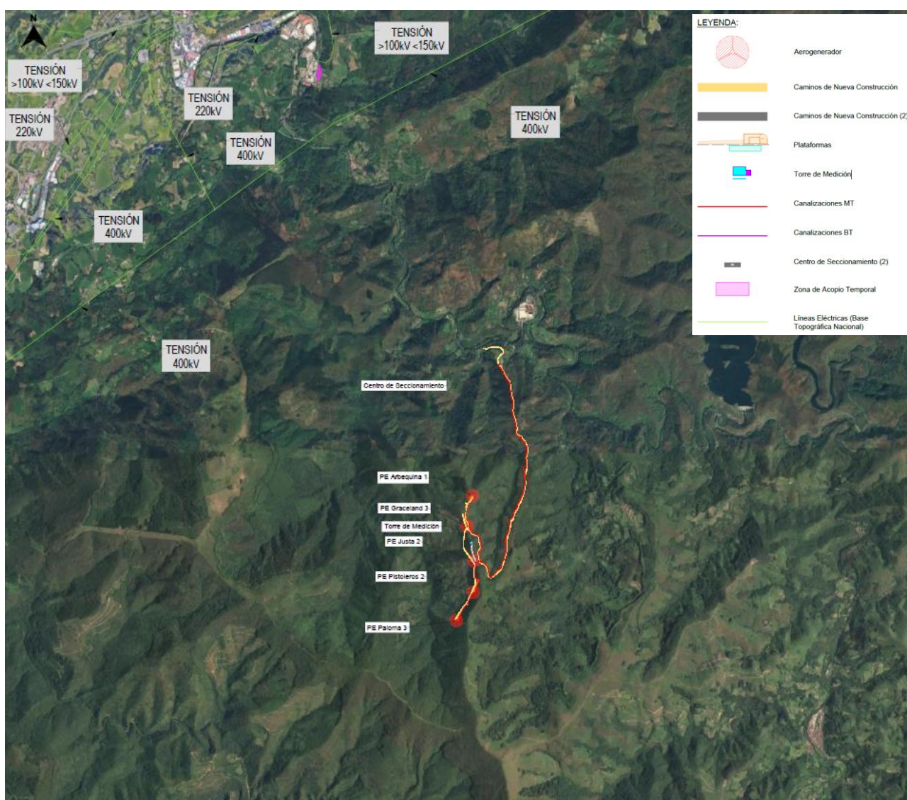
Figura 2. Afecciones del Parque Eólico "PE Ikatz Gane" a Líneas Eléctricas
