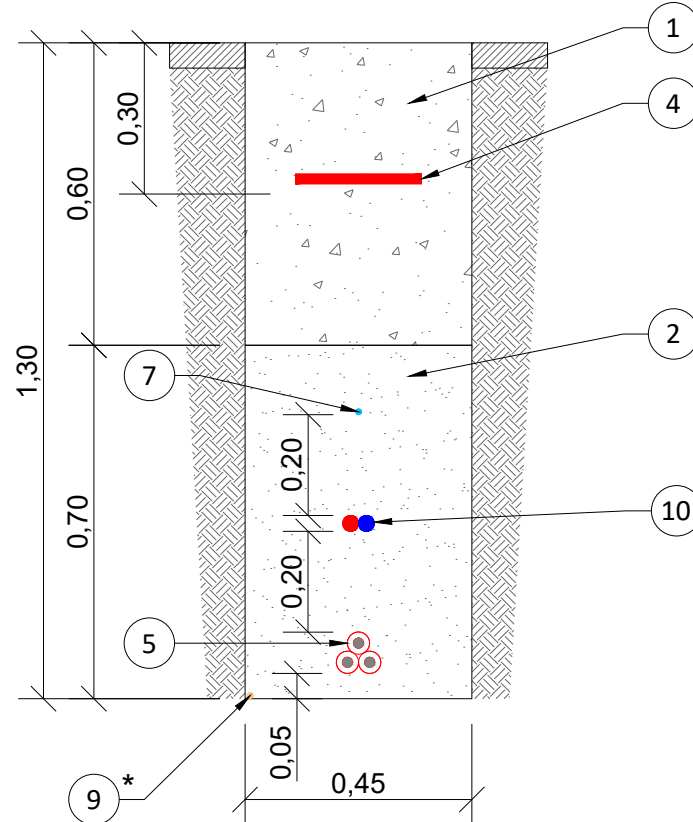
1 LÍNEA, CABLE MT 1 LÍNEA, CABLE BT 1 LÍNEA, CABLE COMUNICACIÓN ENTERRADO DIRECTO
