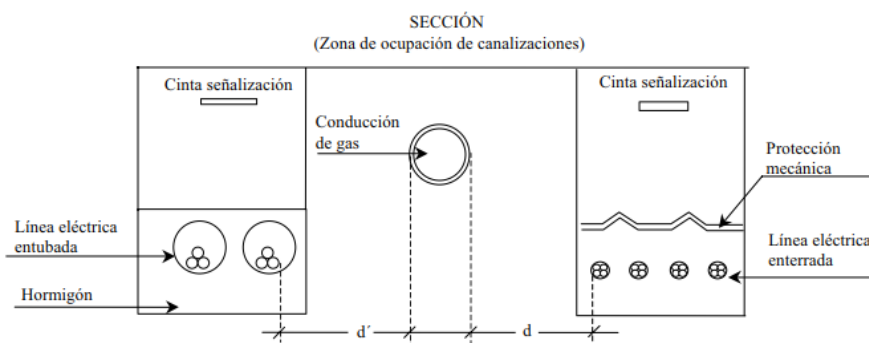
Figura 4: Detalle de paralelismo con canalización de gas
