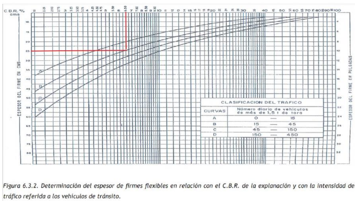
Figura 2: Gráfica de determinación del espesor de firme
