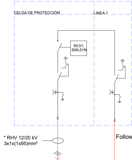
CENTRO DE TRANSFORMACIÓN 1-TST01 2.500 kVA
