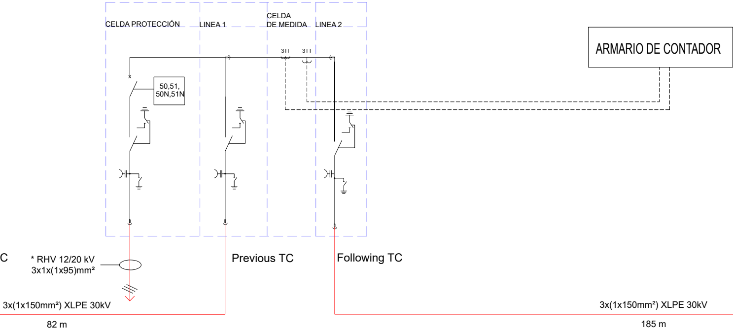
CENTRO DE TRANSFORMACIÓN 2-TST02 2.500 kVA
