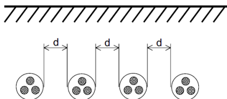
Figura 1. Disposición cable MT.
