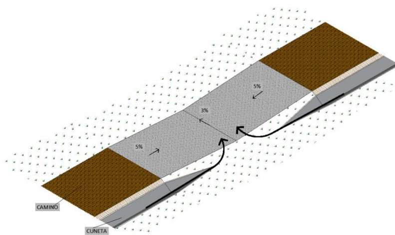
Figura 7: Sección tipo de badén
