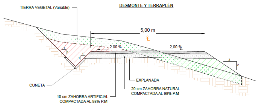
Figura 4: Sección tipo de los viales de acceso
