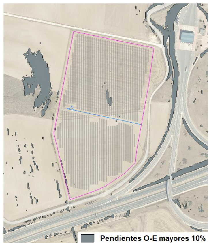
Figura 1 Cálculo de pendientes en la implantación del parque fotovoltaico
