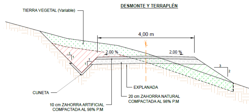
Figura 3: Sección tipo de los viales internos
