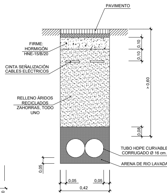
ZANJA A-2 ESCALA 1/10
