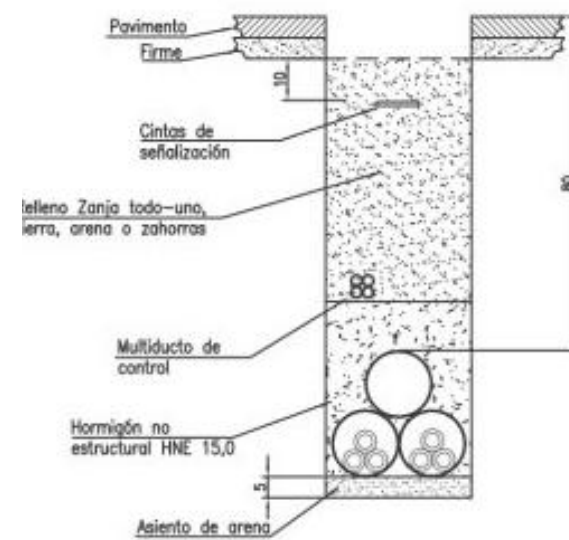
CANALIZACIÓN ENTUBADA EN CALZADA (3 TUBOS 200Ø) COTAS EN CM ESCALA S/E
