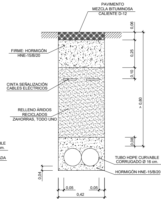
ZANJA C-2 ESCALA 1/10
