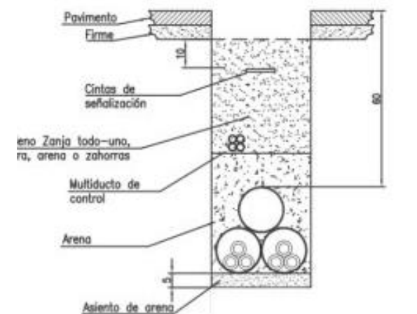
CANALIZACIÓN EN JARDINES O BAJO ACERA (3 TUBOS 200Ø) COTAS EN CM ESCALA S/E
