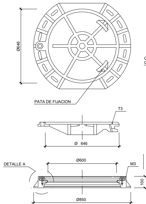
MARCO-TAPA DE FUNDICION M3-T3 (CALZADA) ESCALA 1/10
