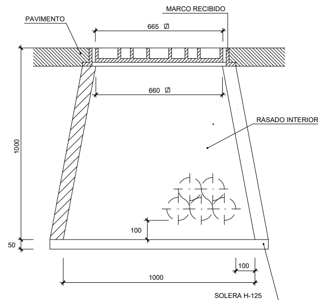
MARCO-TAPA DE FUNDICION M3-T3 (CALZADA) ESCALA 1/10
