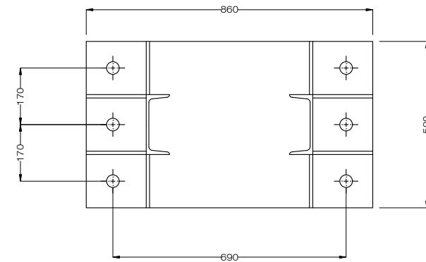
BASE DE POSTE
