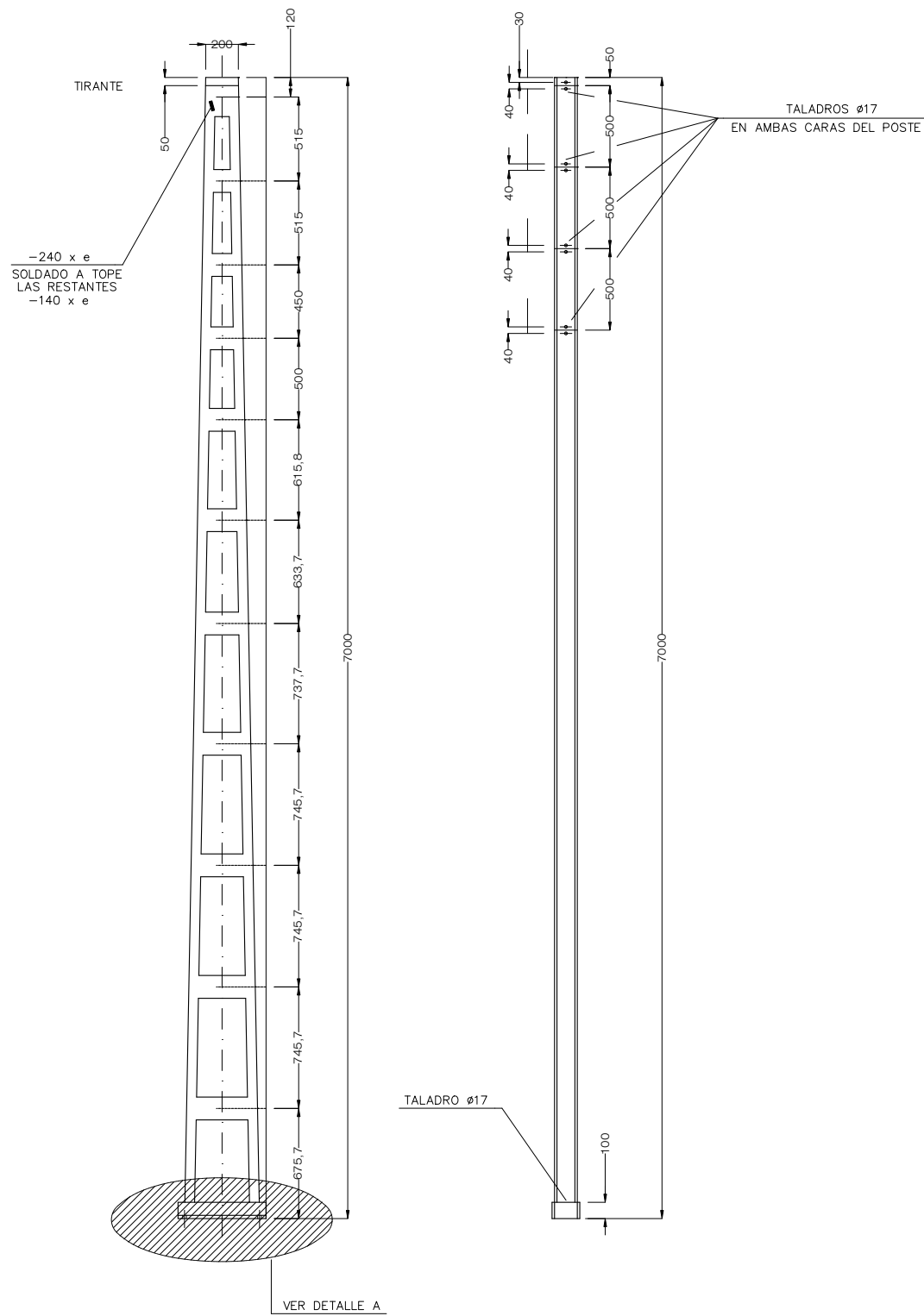
DETALLE DE POSTE X-3
