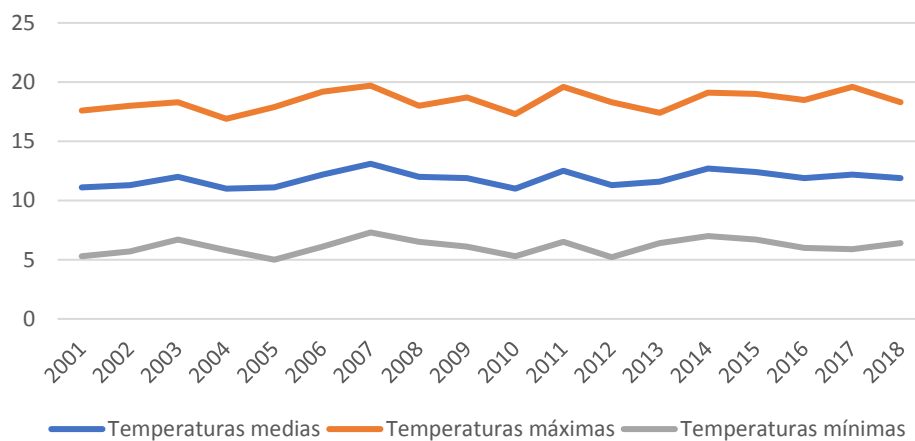
Evolución de la media de temperaturas en Est. Meteo. Gorbea (°C)
