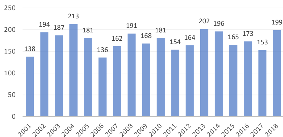
Días de precipitación (2001-2018) en la estación de Iturrieta
