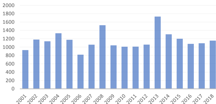
Precipitaciones acumuladas (mm) (2001-2018) en la estación de Iturrieta
