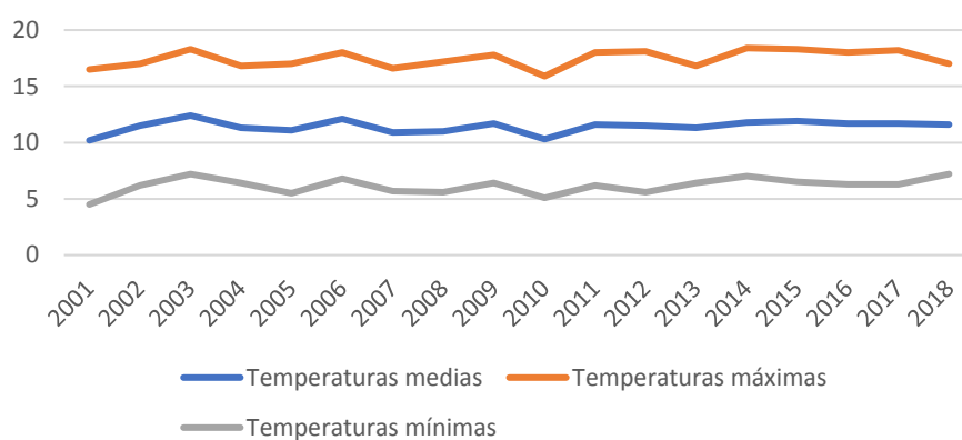
Evolución de la media de temperaturas en Est. Meteo. Arkaute (°C)
