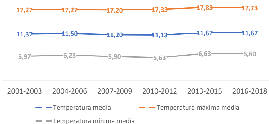
EVOLUCIÓN DE LA MEDIA DE LA TEMPERATURA EN EST. METEO. ARKAUTE
