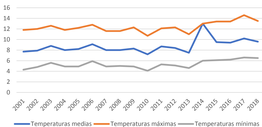
Evolución de la media de temperaturas en Est. Meteo. Herrera (°C)
