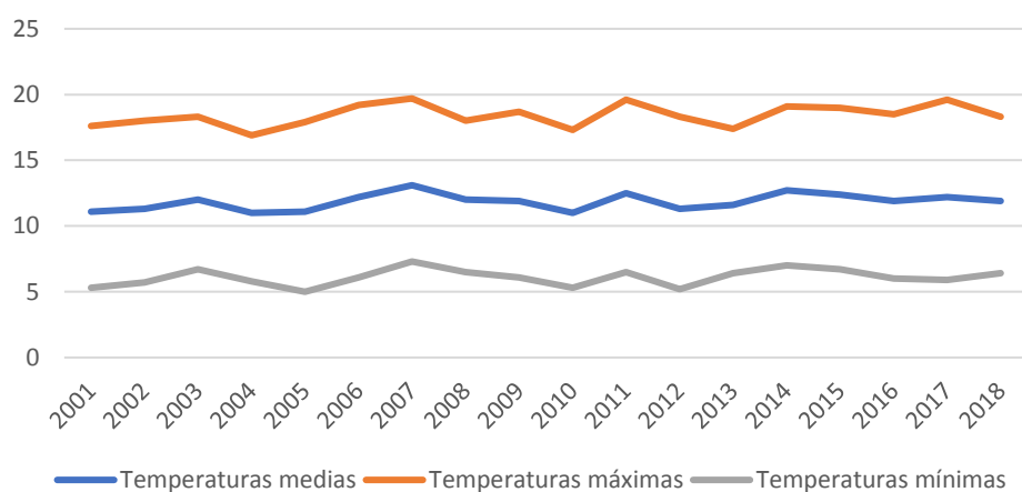
Evolución de la media de temperaturas en Est. Meteo. Espejo (°C)
