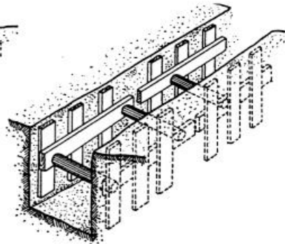
ENTIBACIÓN SEMICUAJADA
