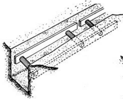
ENTIBACIÓN LIGERA
