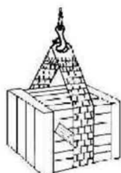
Eslinga simple Eslinga sin fin Eslinga para lazada Eslinga de 2 ramales Eslinga de 4 ramales
