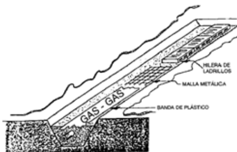
FORMAS MÁS USUALES DE SEÑALIZACIÓN INTERIOR Y PROTECCIÓN EMPLEADAS EN CONDUCCIONES DE GAS
