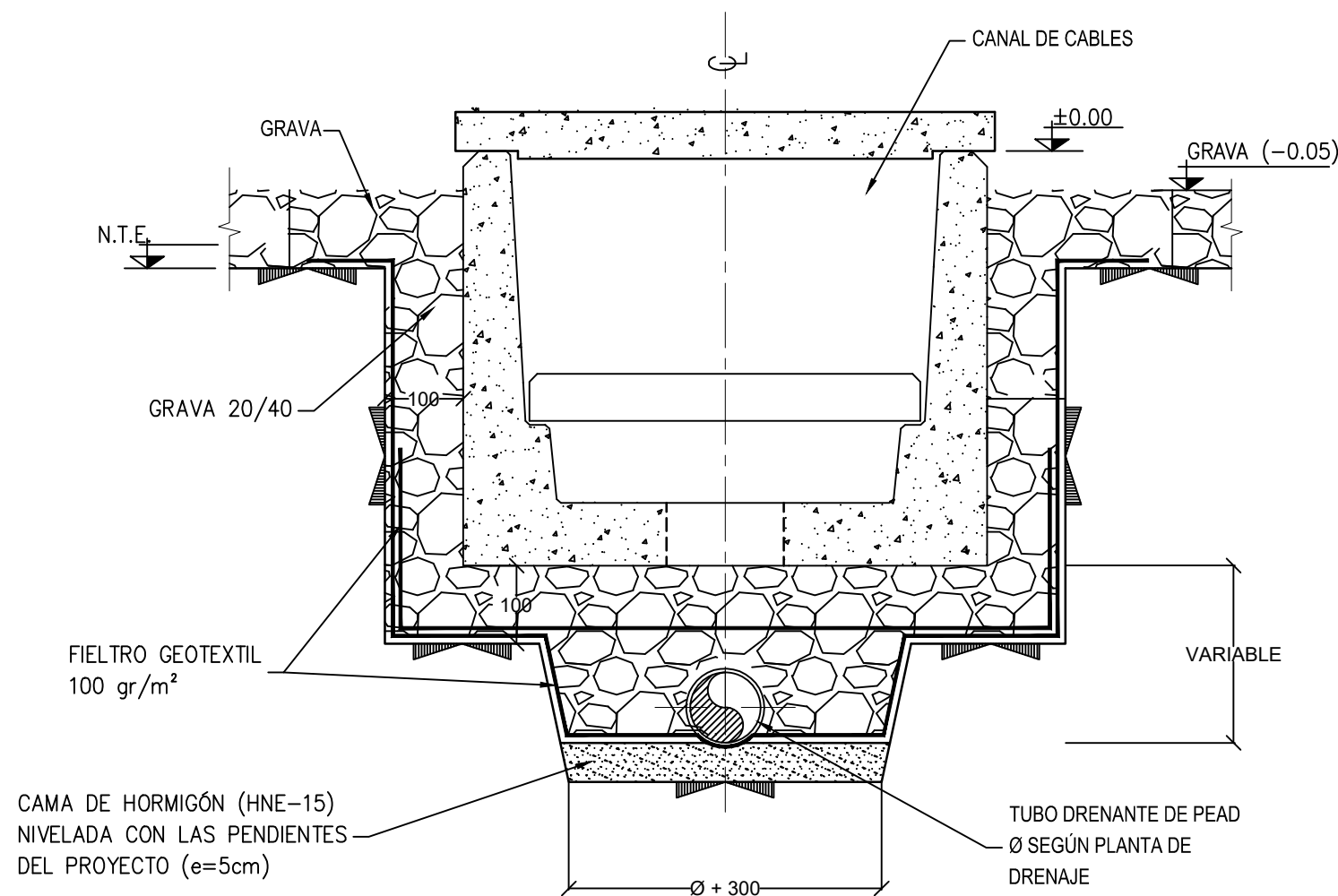
SECCIÓN TIPO
