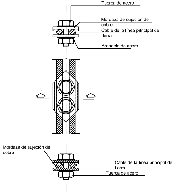
DETALLE A
