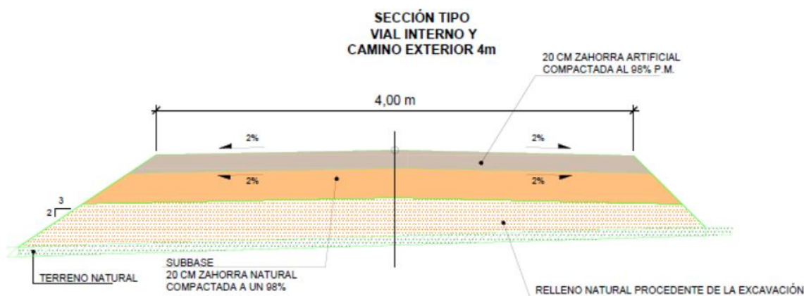
Imagen 4. Ejemplo de sección tipo vial interno y camino exterior de 4 m
