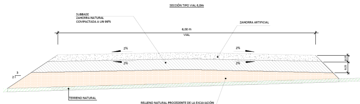
Imagen 5. Ejemplo de sección tipo vial acceso de 6 m
