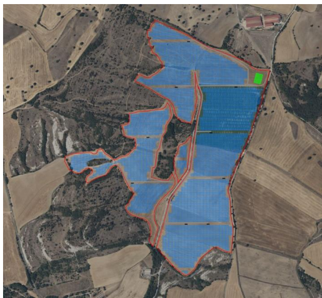
Imagen 1. Plano de situación de la planta FV
