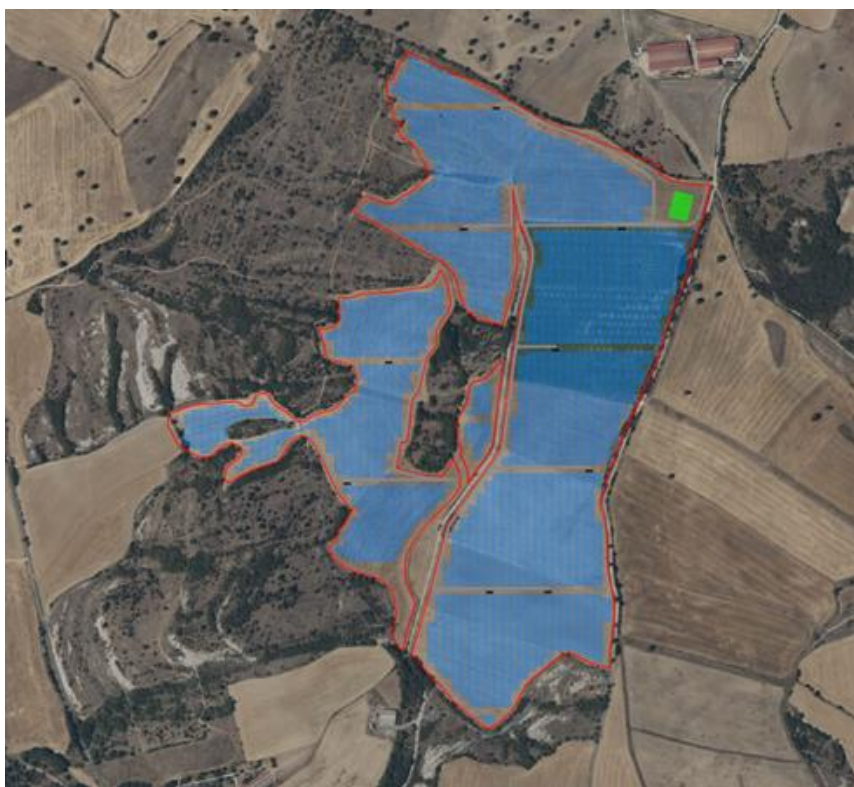
Imagen 2. Layout planta FV
