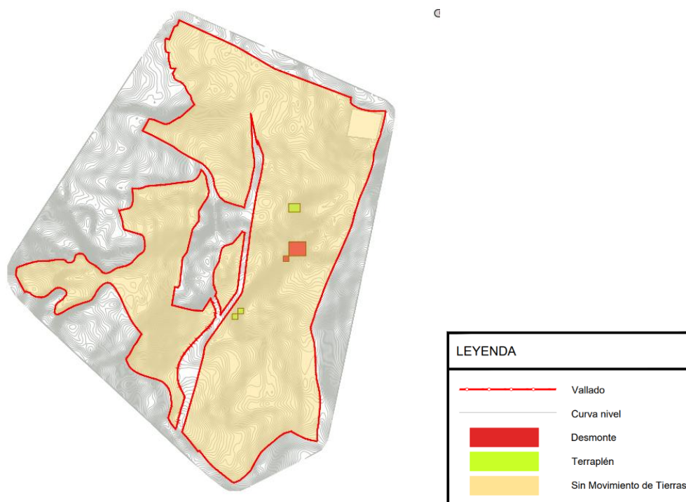
Plano de Movimiento de tierras
