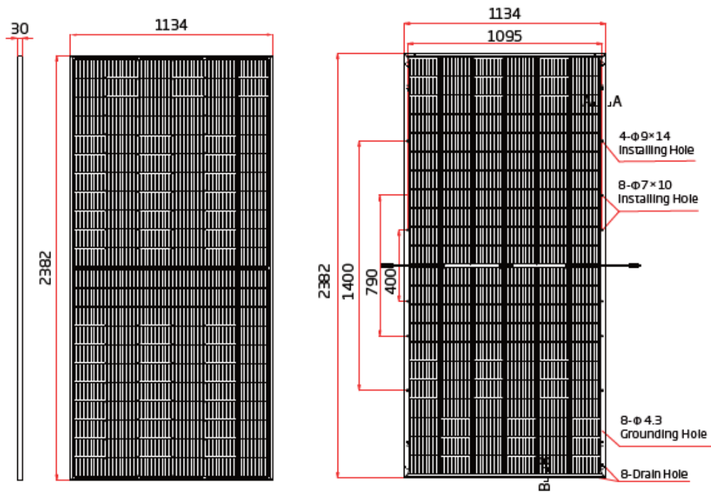
Imagen 3. Módulo FV 620 Wp
