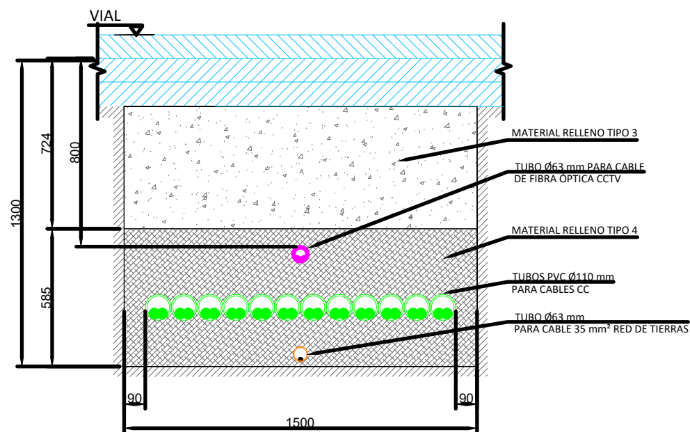
SECCIÓN A-A
