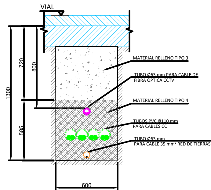
SECCIÓN A-A
