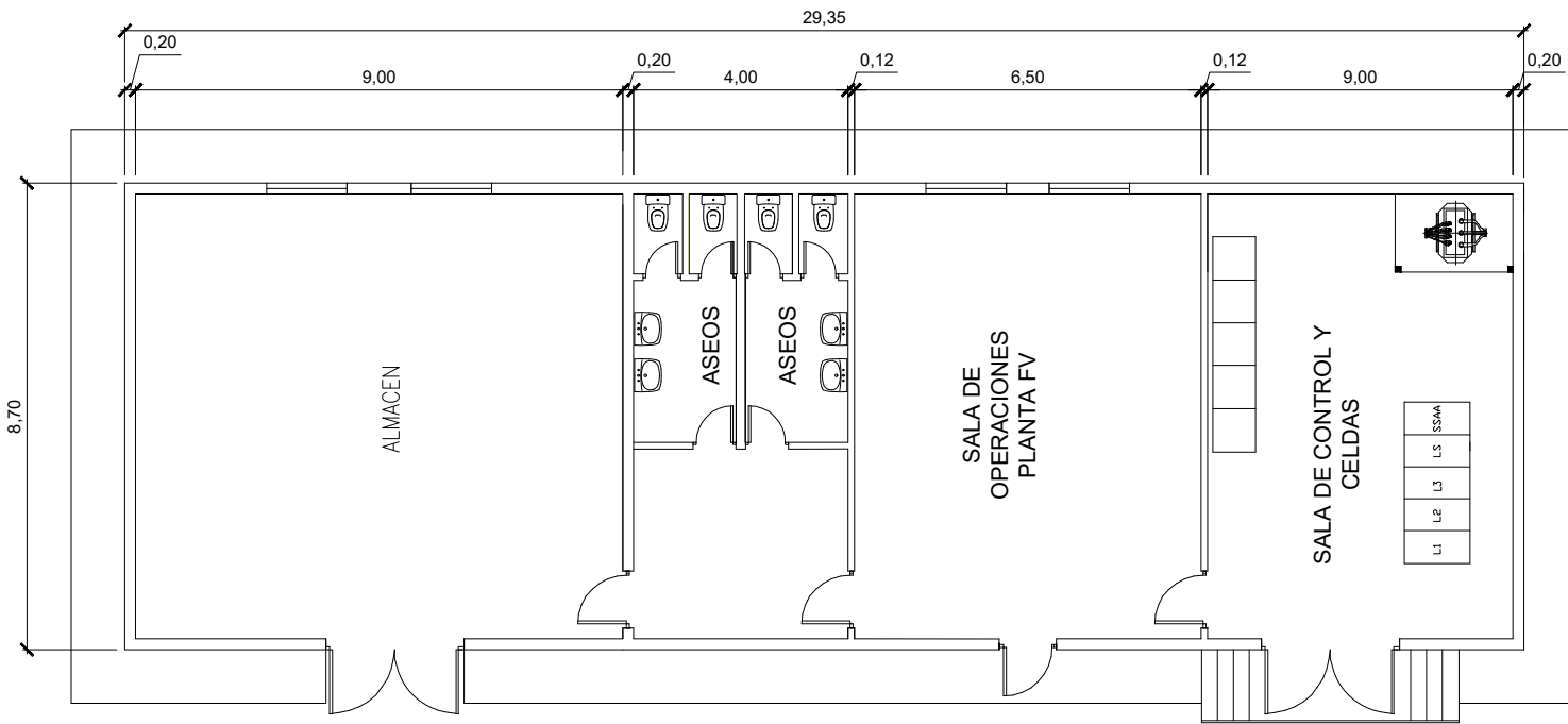
PLANTA Esc: 1:150
