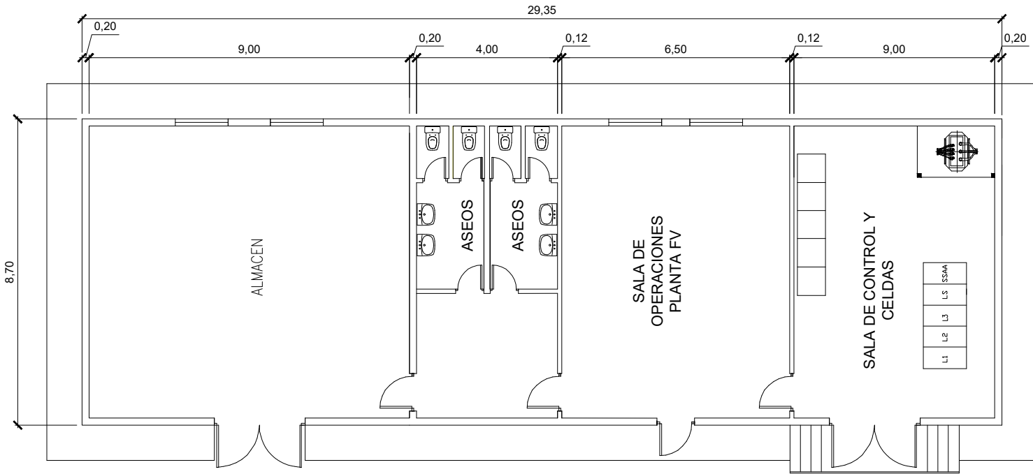
PLANTA Esc: 1:150
