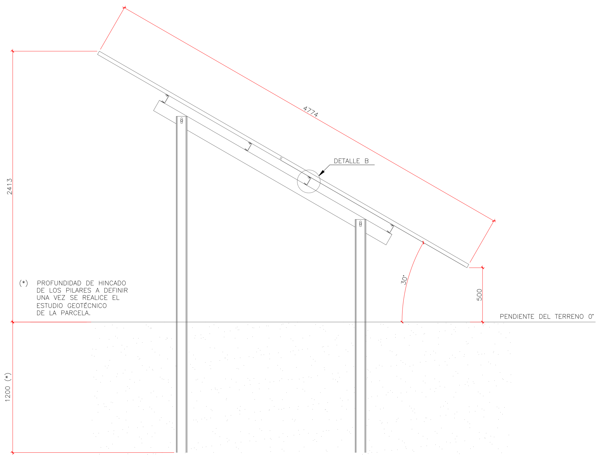
PERFIL S/E
