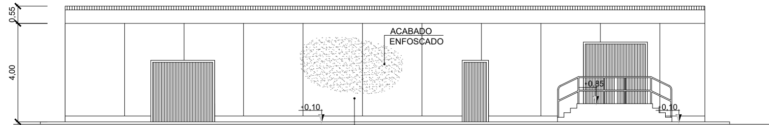
PANEL DE FACHADA PREFABRICADO DE HORMIGÓN ARMADO CON AISLAMIENTO ALZADO "A" Esc: 1:150
