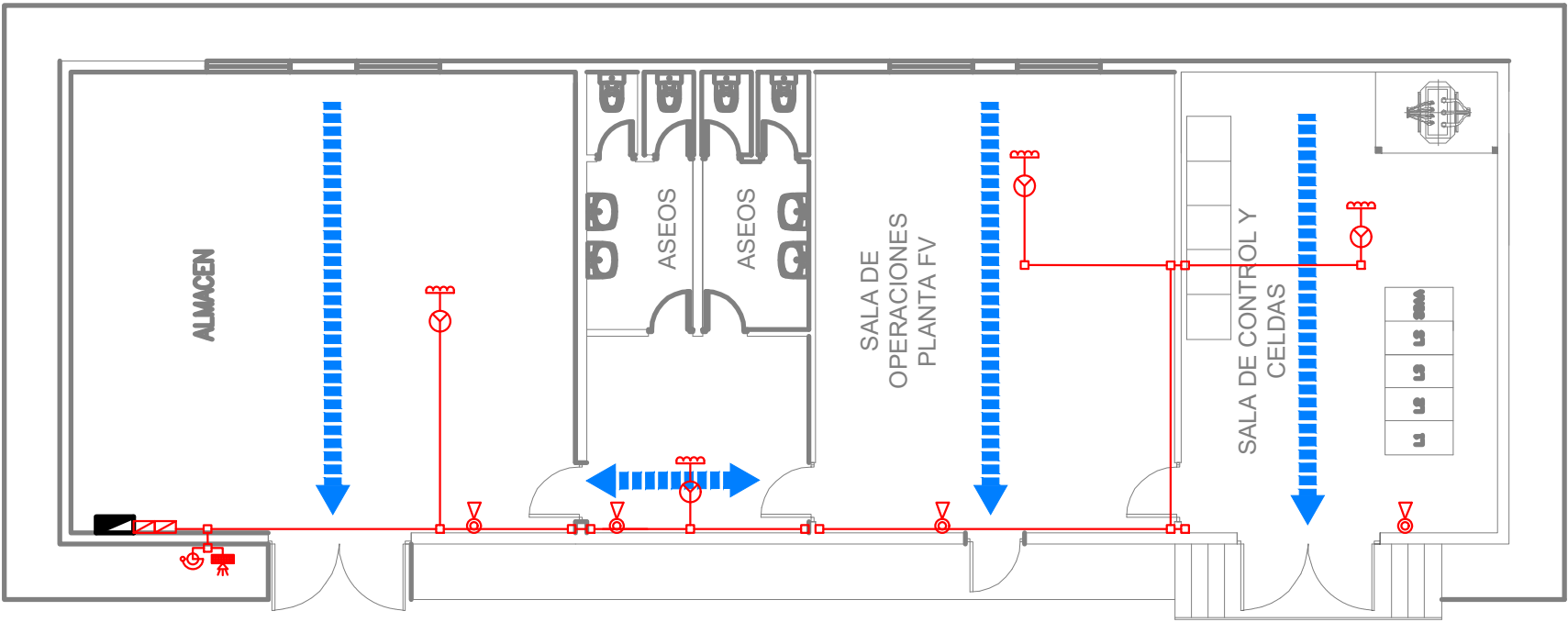
PLANTA Esc: 1:125
