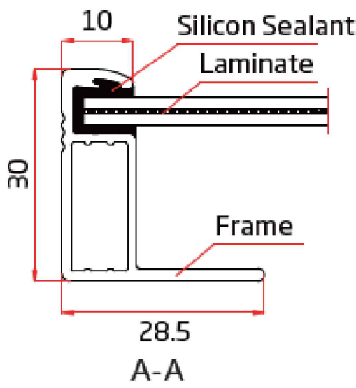
A-A
