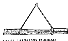
CARGA LARGA (DOS ESLINGAS)
