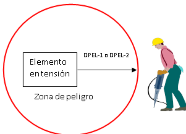
Imagen 2. Respeto de la zona de peligro de trabajo para trabajos próximos a elementos en tensión.
