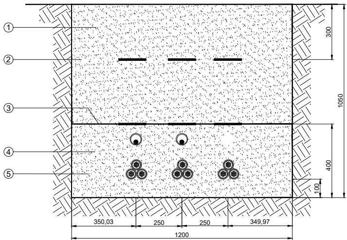
ZANJA DIRECTAMENTE ENTERRADA 3 TERNAS
