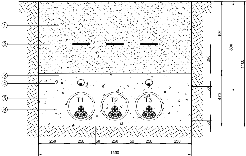
ZANJA ENTUBADA HORMIGONADA 3 TERNAS TUBO Ø250mm
