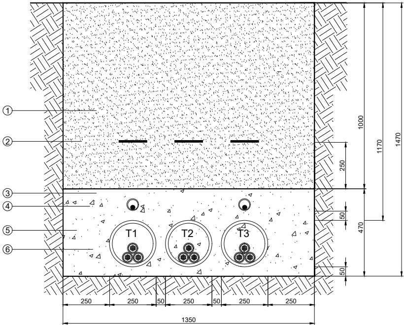
ZANJA ENTUBADA HORMIGONADA EN TERRENO DE CULTIVO 3 TERNAS TUBO Ø250mm
