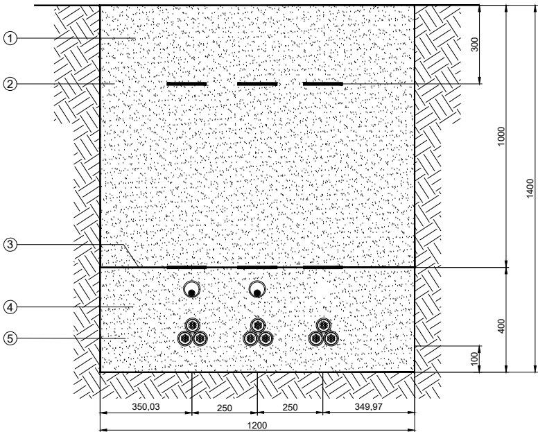
ZANJA DIRECTAMENTE ENTERRADA EN TERRENO DE CULTIVO 3 TERNAS
