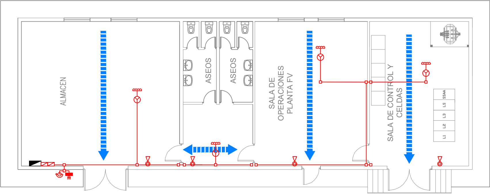
PLANTA Esc: 1:125
