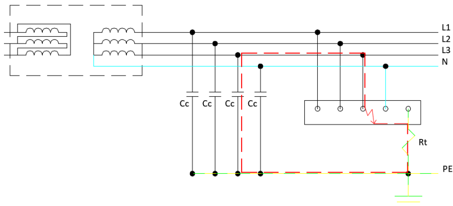
Bucle de falta a tierra en sistema con nuestro aislado
