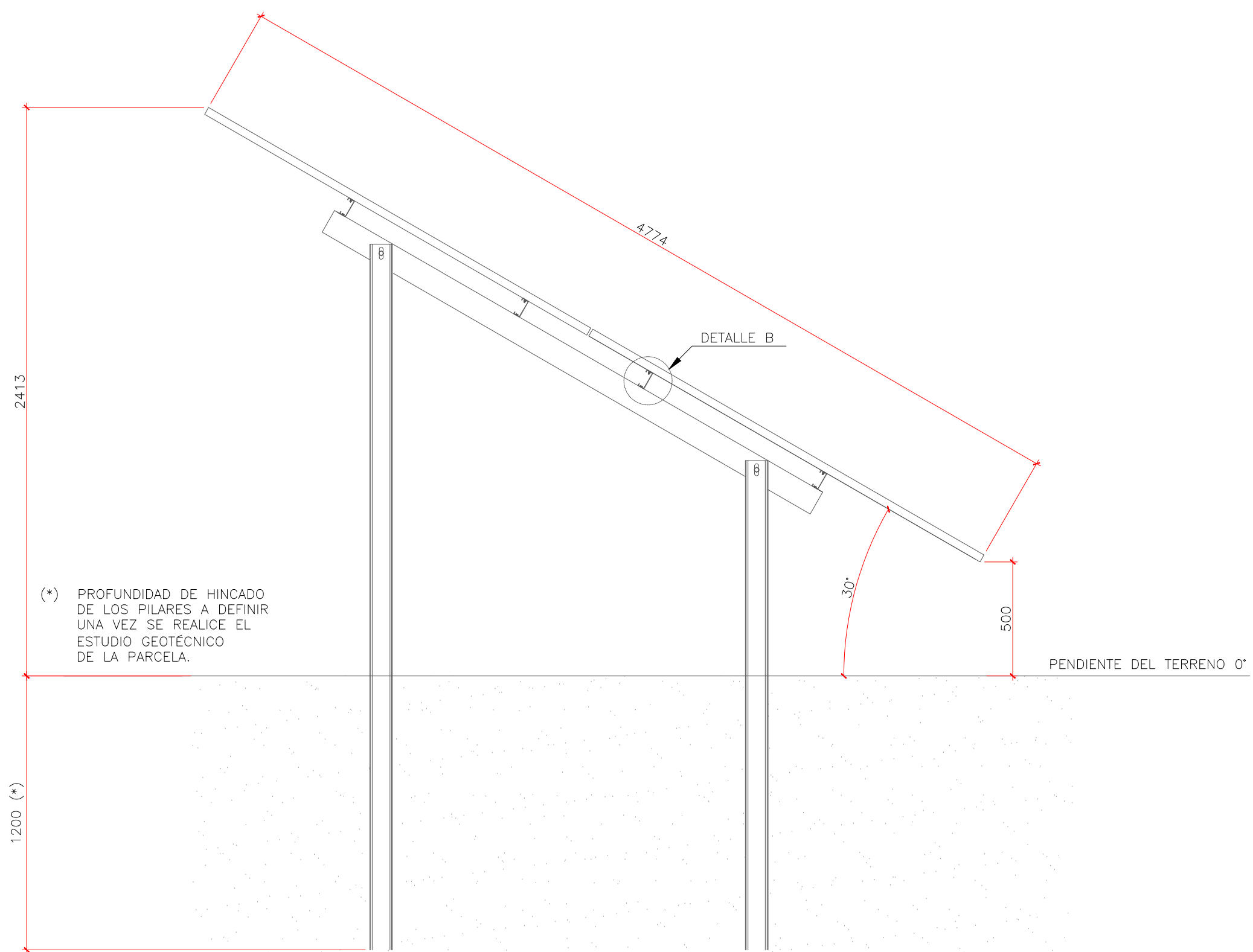
PERFIL S/E
