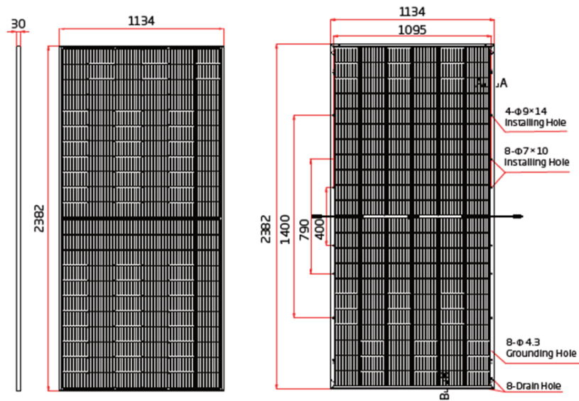
Imagen 4. Módulo FV ¡Error! No se encuentra el origen de la referencia. Wp
