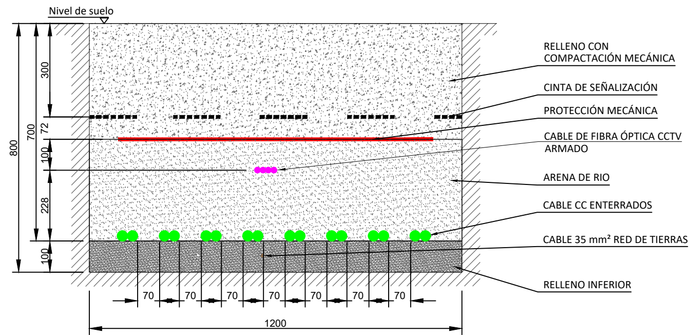
ZANJA BAJA TENSIÓN CORRIENTE CONTINUA 7 circuitos Al 2x1x400 mm 2 (CC) + circuitos FO + Cable red de tierra Cu desnudo 50 mm 2
