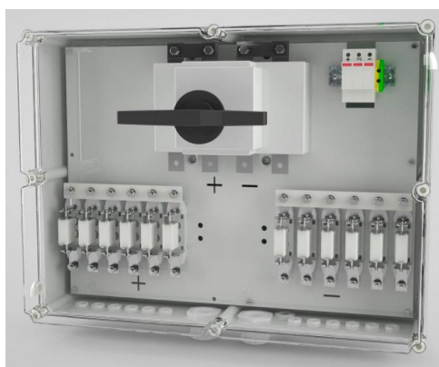
Imagen 5. Ejemplo de caja de nivel 1
