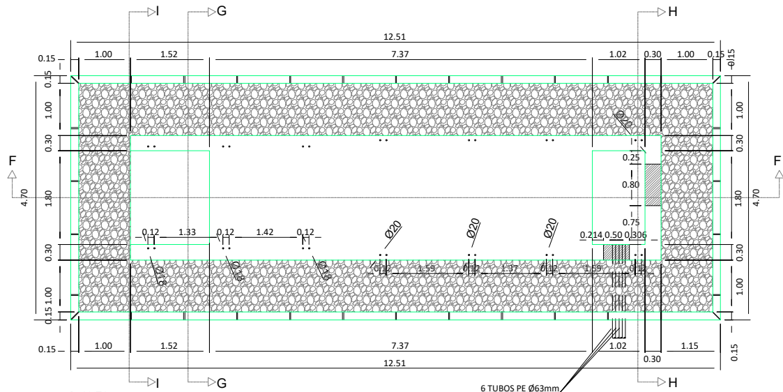
PLANTA Escala 1:40
