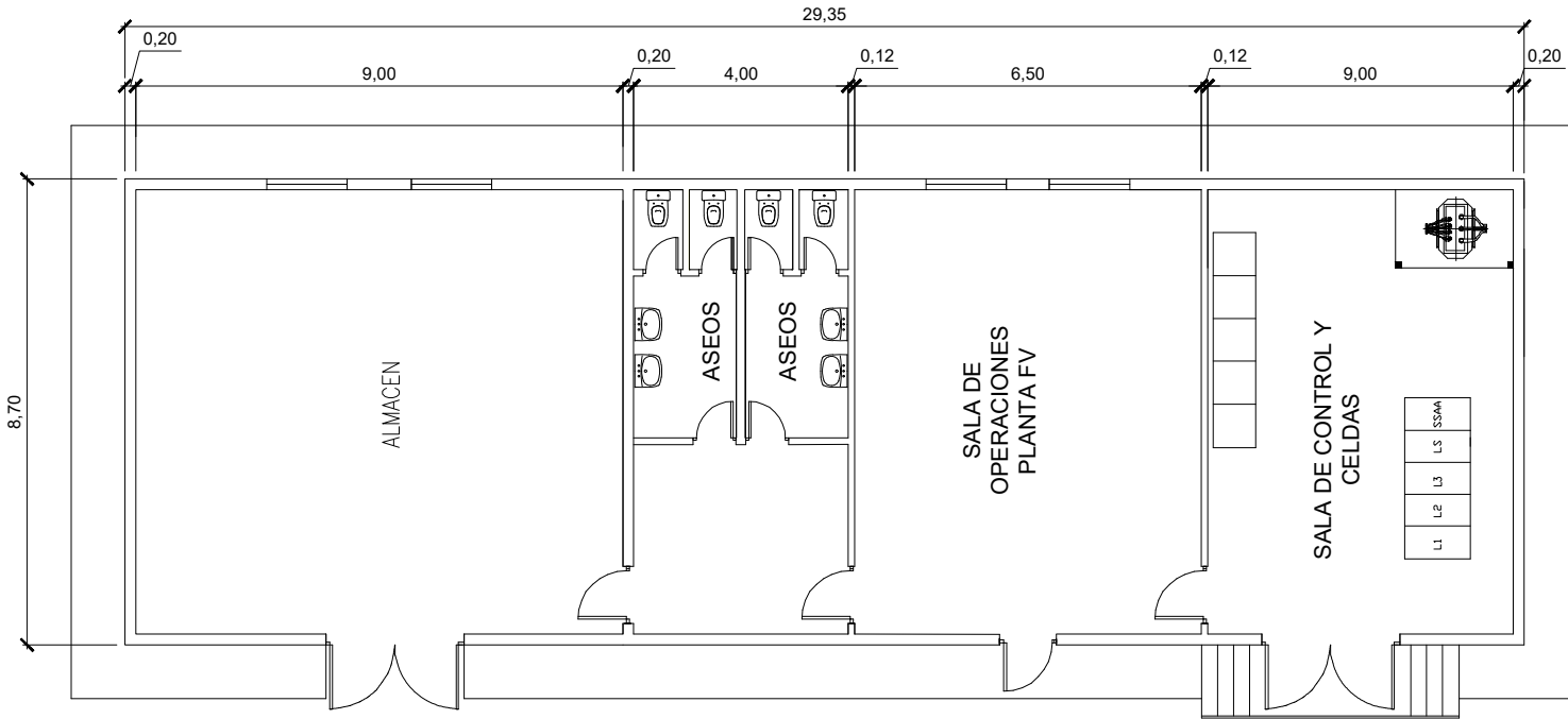
PLANTA Esc: 1:150
