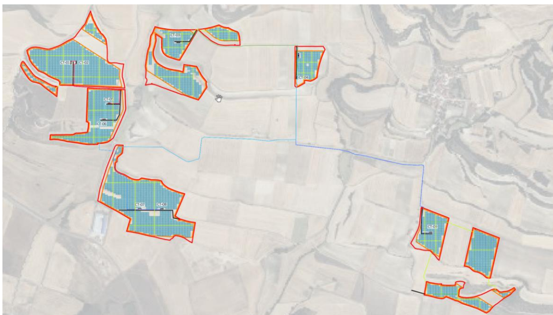
Imagen 3. Layout planta FV
