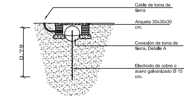
ALZADO - SECCIÓN
