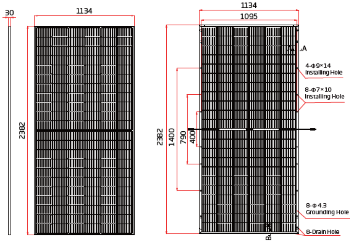
Imagen 4. Módulo FV 620 Wp
