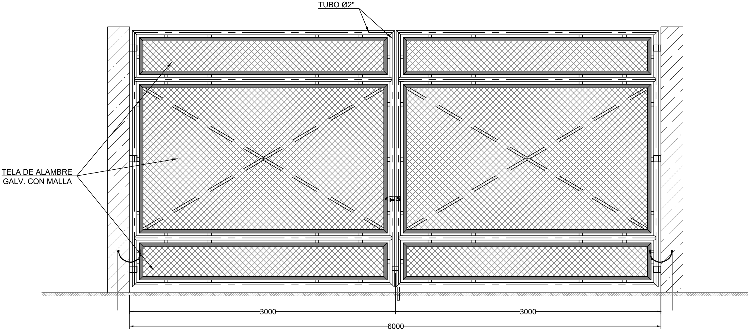
PUERTA PARA VEHÍCULOS
