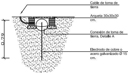
ALZADO - SECCIÓN
