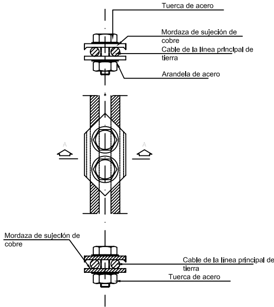
DETALLE A
