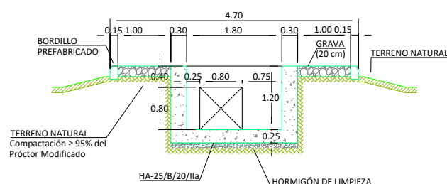
SECCIÓN H-H Escala 1:40
