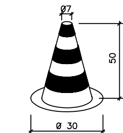
CONO BALIZAMIENTO
