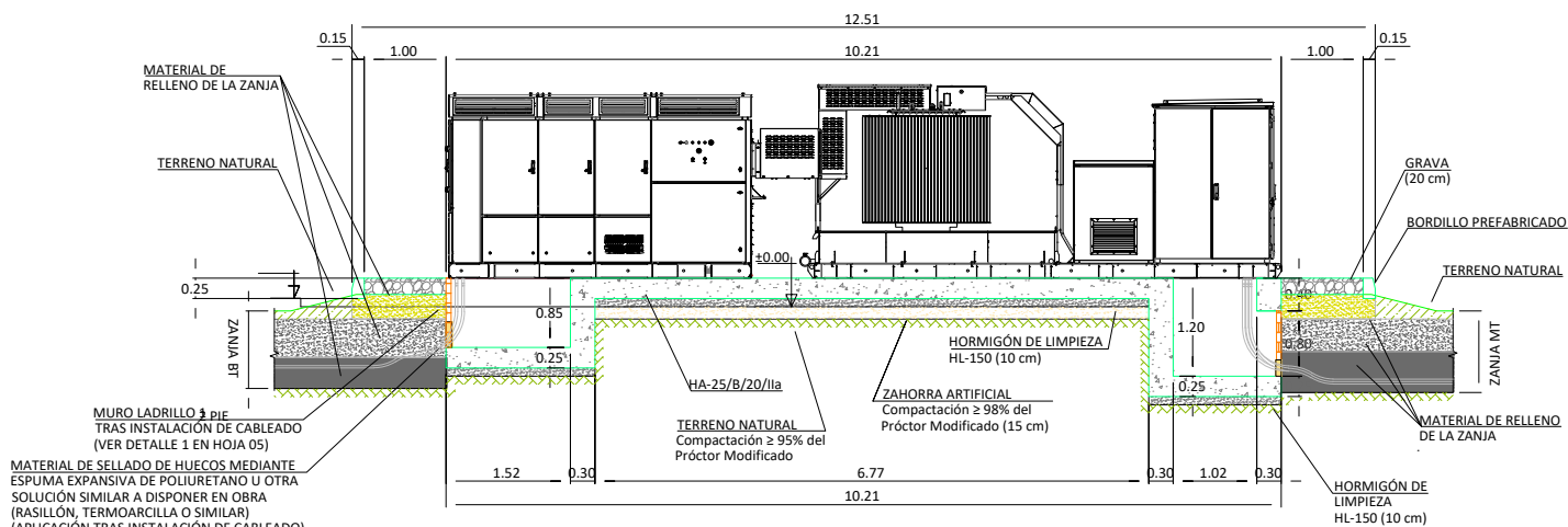
SECCIÓN F-F Escala 1:40
