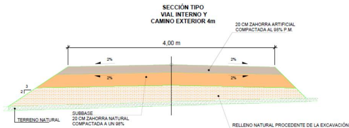
Imagen 10. Ejemplo de sección tipo vial interno y camino exterior de 4 m
