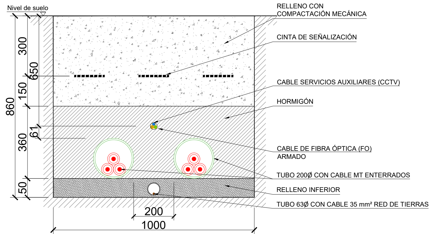
ZANJA MEDIA TENSIÓN BAJO CAMINO Hasta 2 circuitos Al 3x1x630/240/150 mm² (MT) + circuitos FO + circuito SSAA - CCTV + Cable red de tierra Cu desnudo 35 mm²
