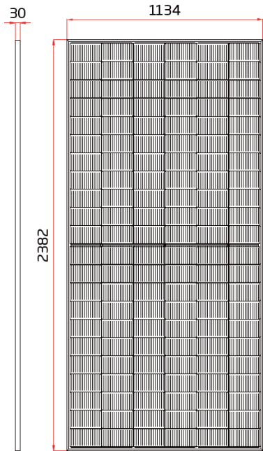
Imagen 4. Módulo FV 620 Wp
