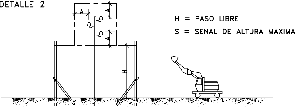
DETALLE 2
