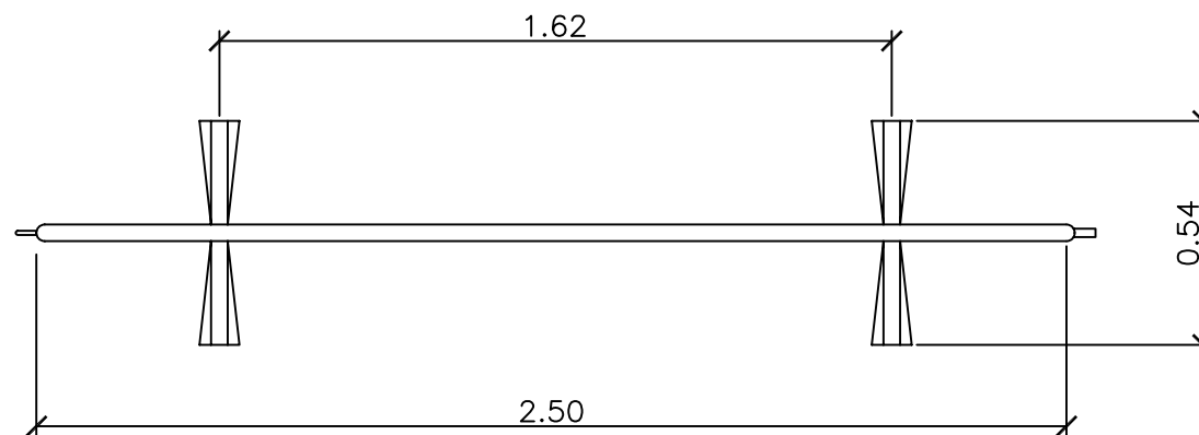
PLANTA
