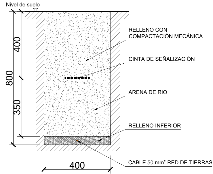
ZANJA TIERRA CENTRO DE TRANSFORMACIÓN Cable red de tierra Cu desnudo 50 mm²
