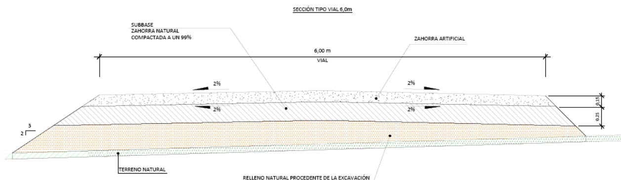
Imagen 11. Ejemplo de sección tipo vial acceso de 6 m
