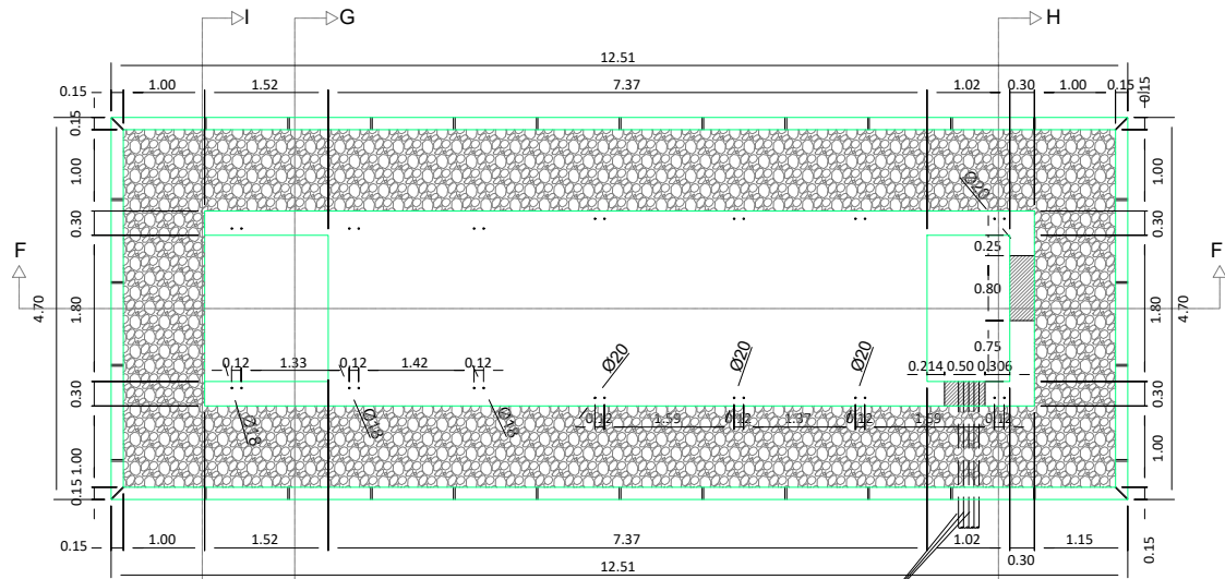
PLANTA Escala 1:40
