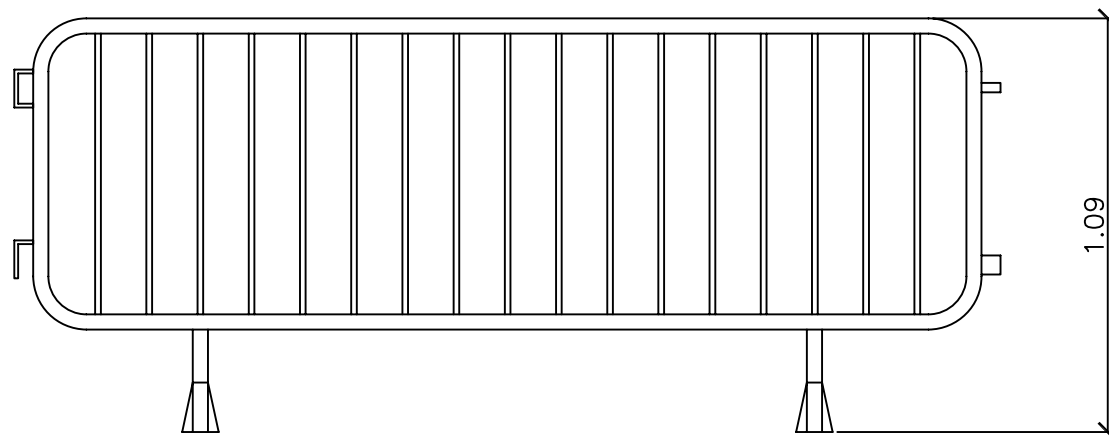
ALZADO
