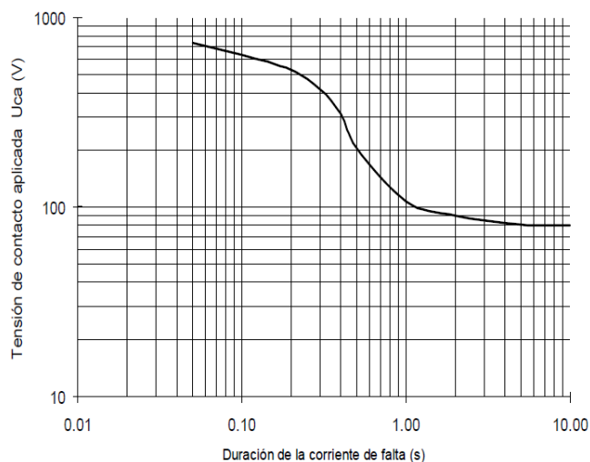
Máxima tensión de contacto admisible en función de la duración de la falta
