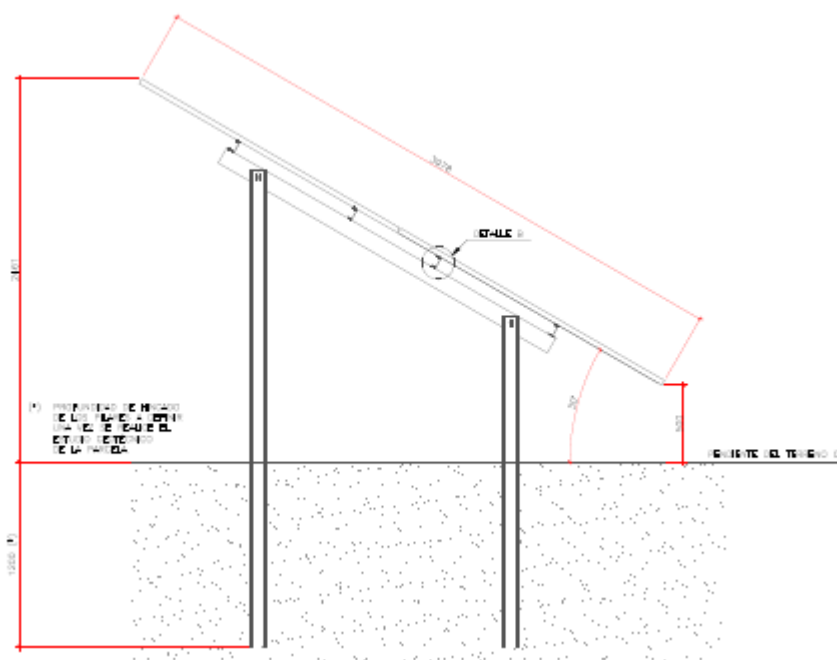
Cimentación estructura fija 2V
