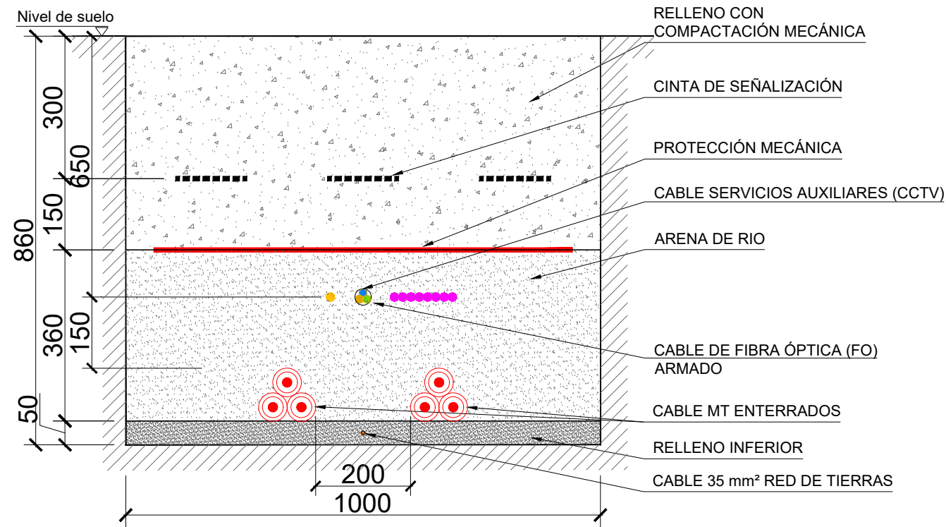
ZANJA MEDIA TENSIÓN Hasta 2 circuitos Al 3x1x630/240/150 mm² (MT) + circuitos FO + circuito SSAA - CCTV + Cable red de tierra Cu desnudo 35 mm²
