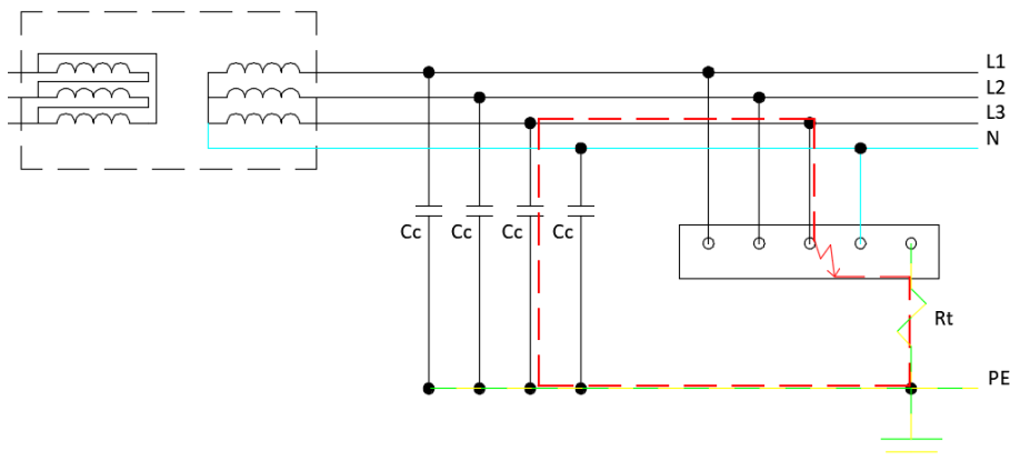
Bucle de falta a tierra en sistema con neutro aislado
