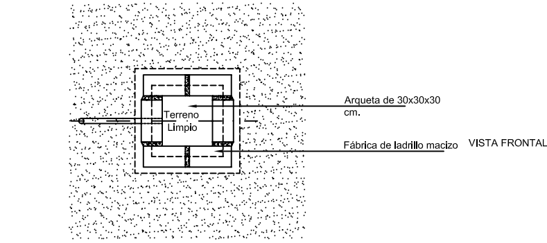
TOMA DE TIERRA NORMALIZADA GENERAL DE LA OBRA RESISTENCIA 80 OHMIOS, RESISTIVIDAD 50 M. OHMIOS TOMA TIERRA
