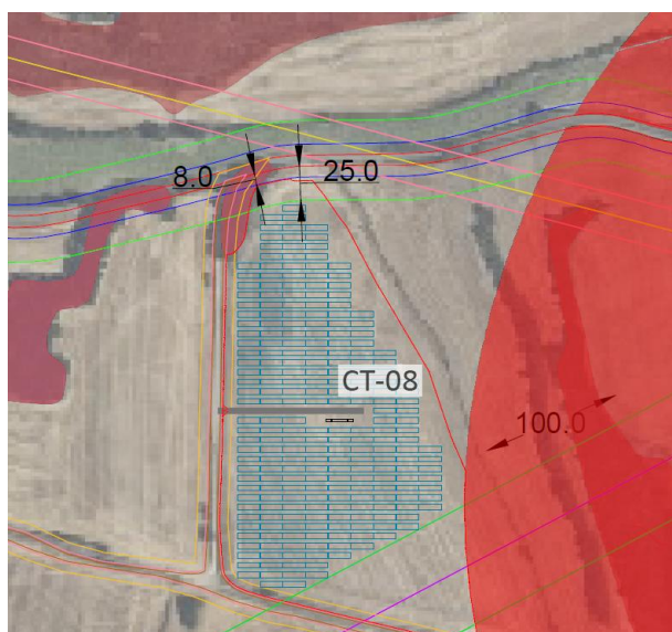
Imagen 7. Detalle A-4325
