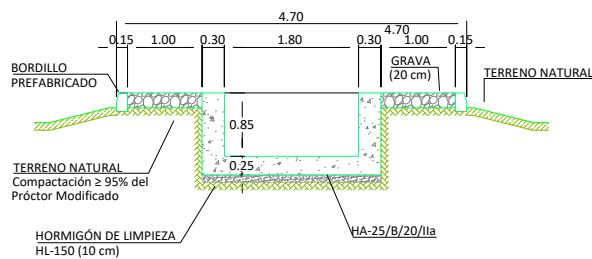
SECCIÓN G-G Escala 1:40
