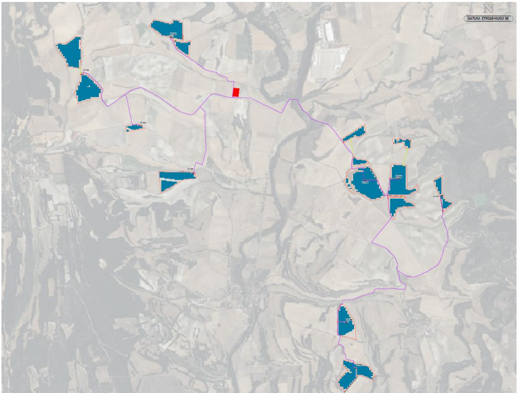
Imagen 3. Layout planta FV
