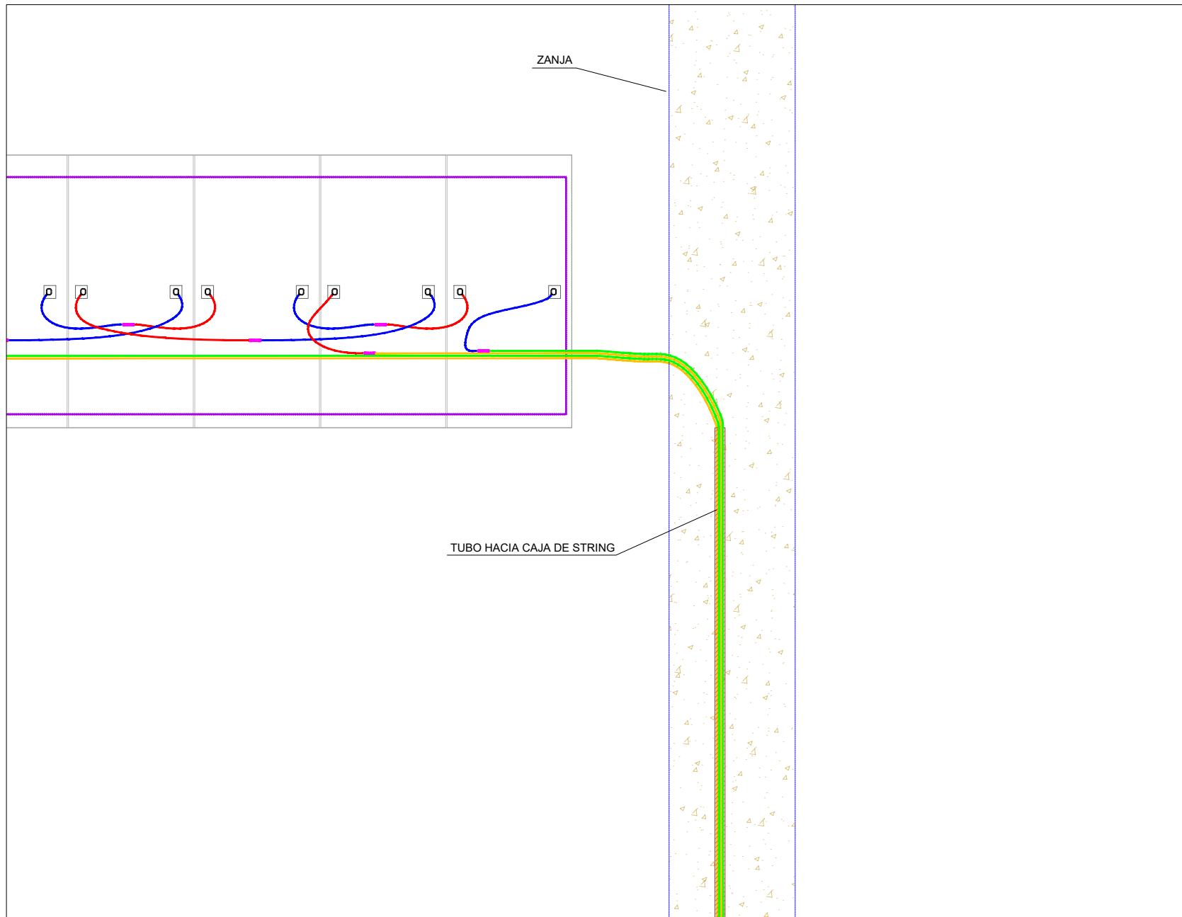
REPRESENTACIÓN ESQUEMÁTICA DEL CONEXIONADO DE MÓDULOS EN UN SEGUIDOR
