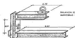
TRASLADOS DE TUBOS
