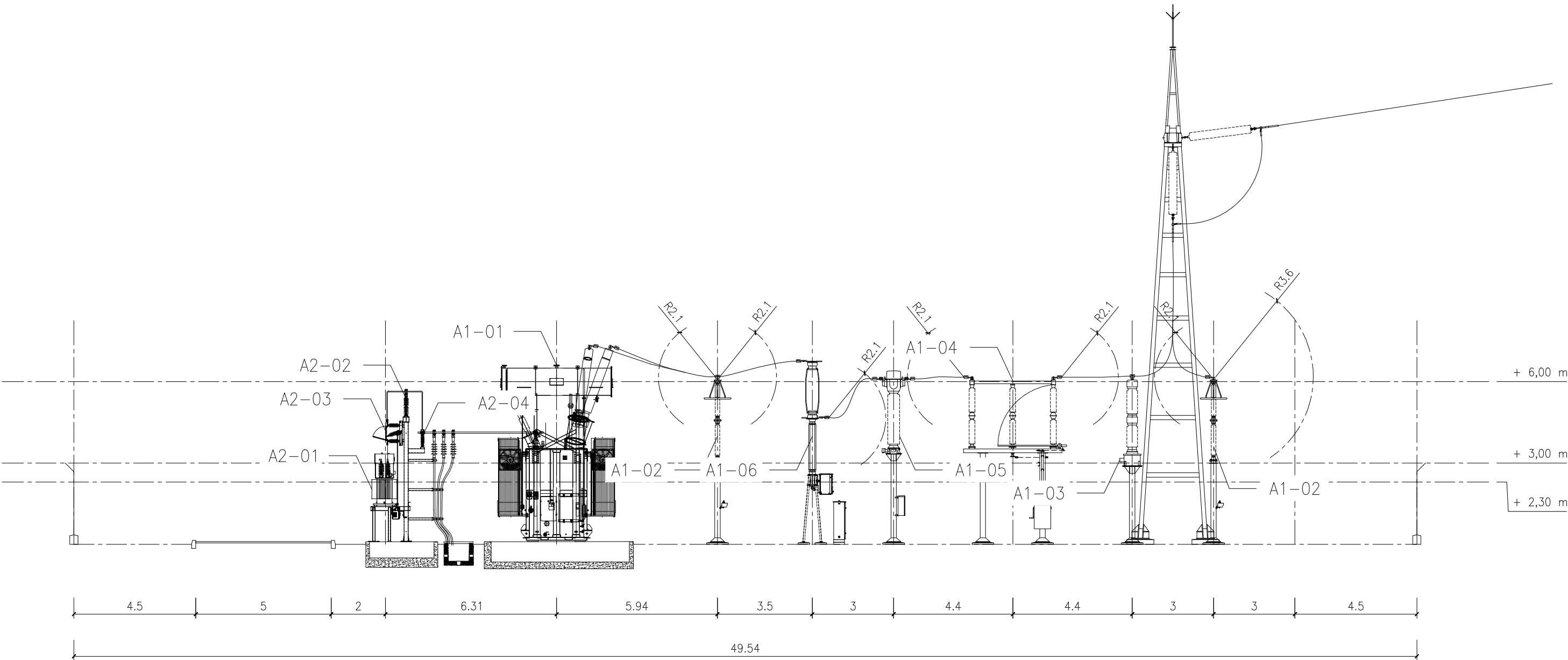
SECCIÓN A-A
