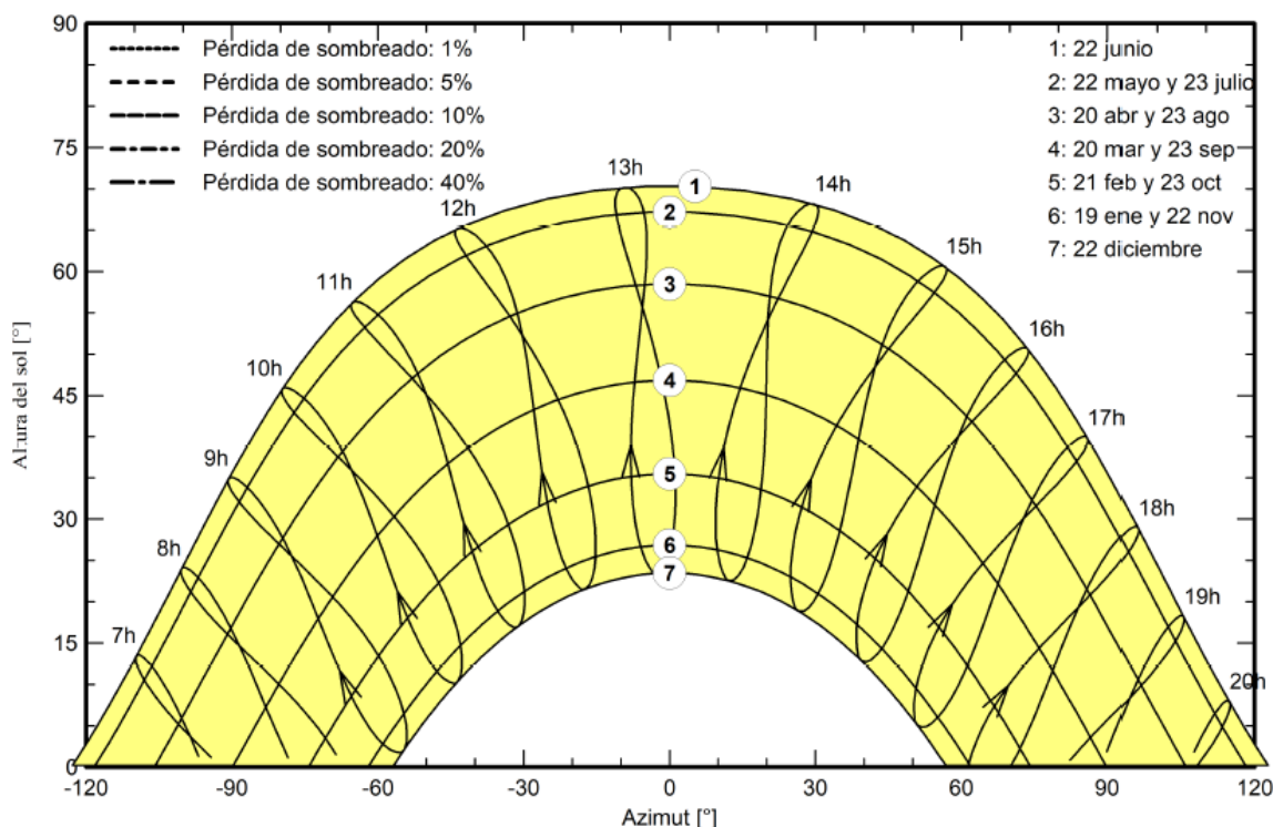
Ilustración 6 : Perfil del horizonte
