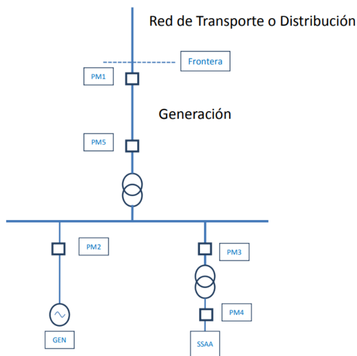
Ilustración 12:Esquema Tipo 1 según Apéndice A de TEC/128/2019
