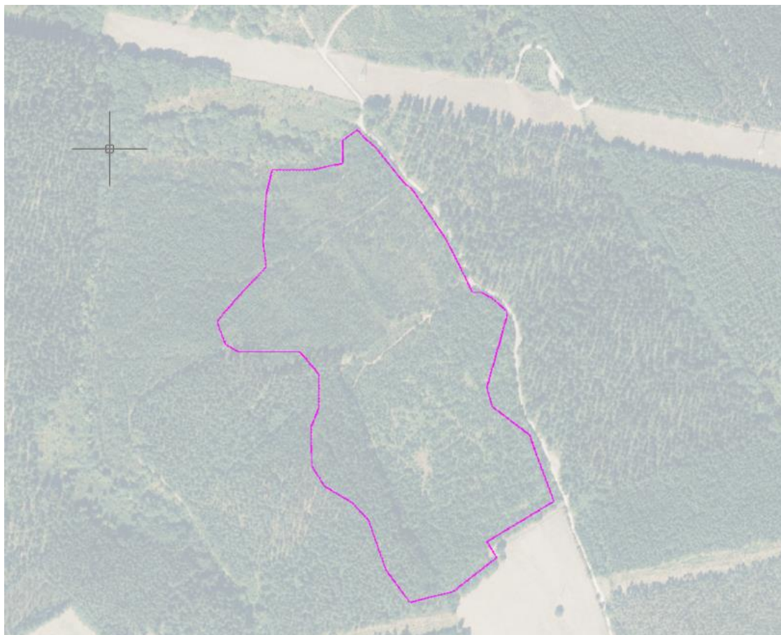
Ilustración 4 : Superficie instalación.
