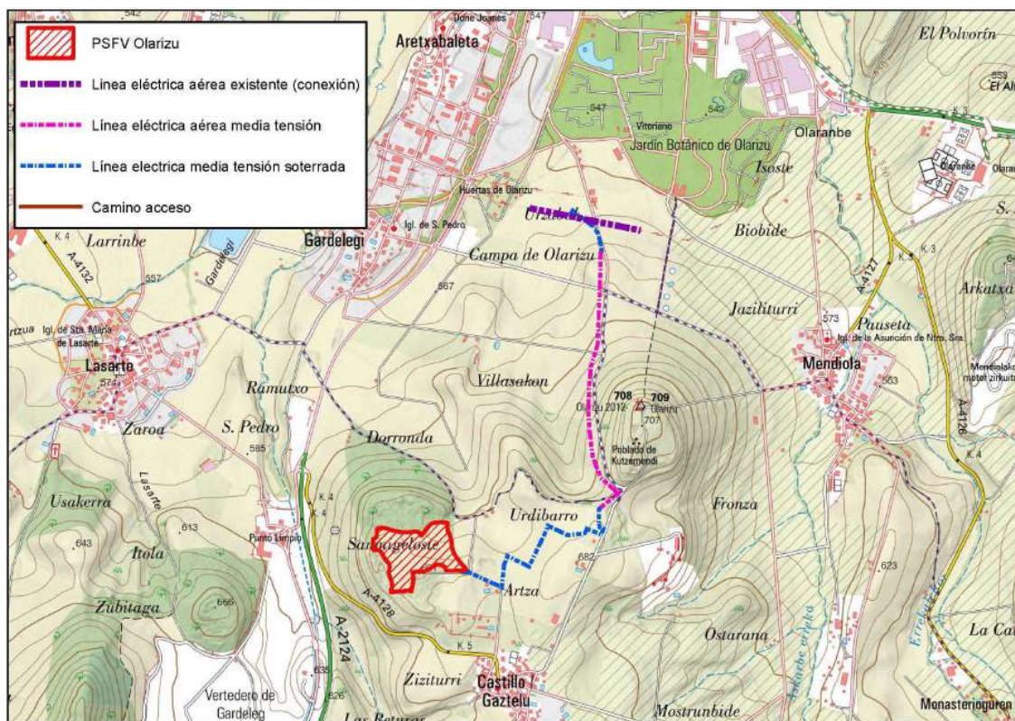
Imagen 4. Implantación del proyecto sobre topográfico
