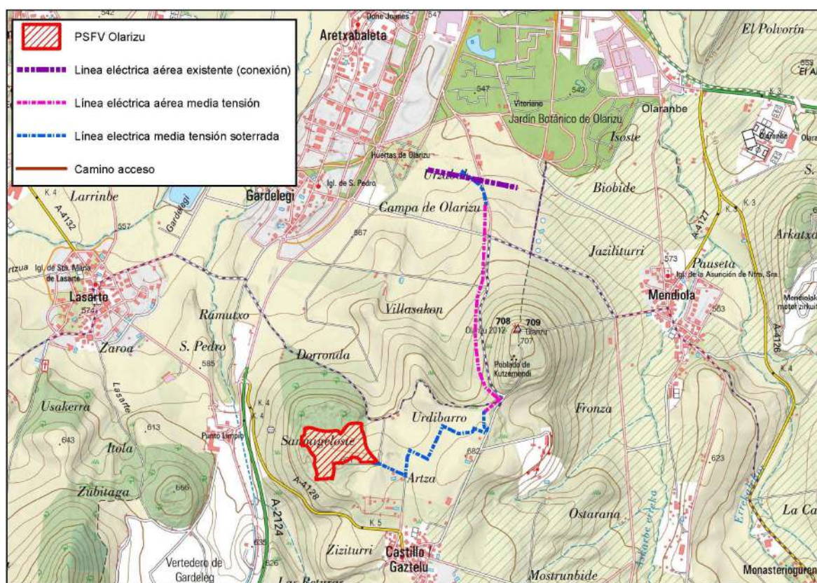
Imagen 2. Implantación de la PSFV Olarizu seleccionada tras el estudio de alternativas
