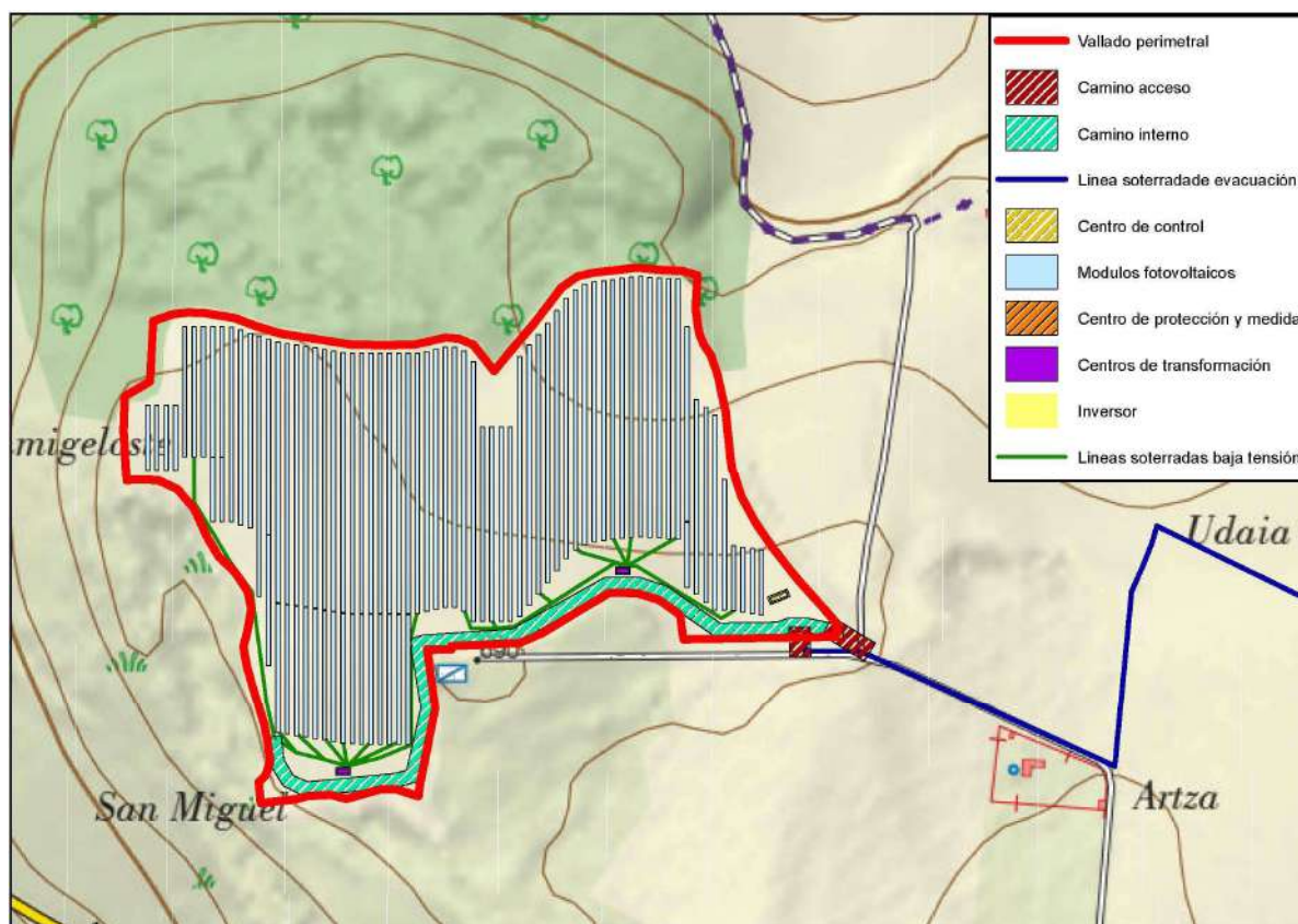
Imagen 6. Detalle de la Implantación de la PSFV sobre ortofoto
