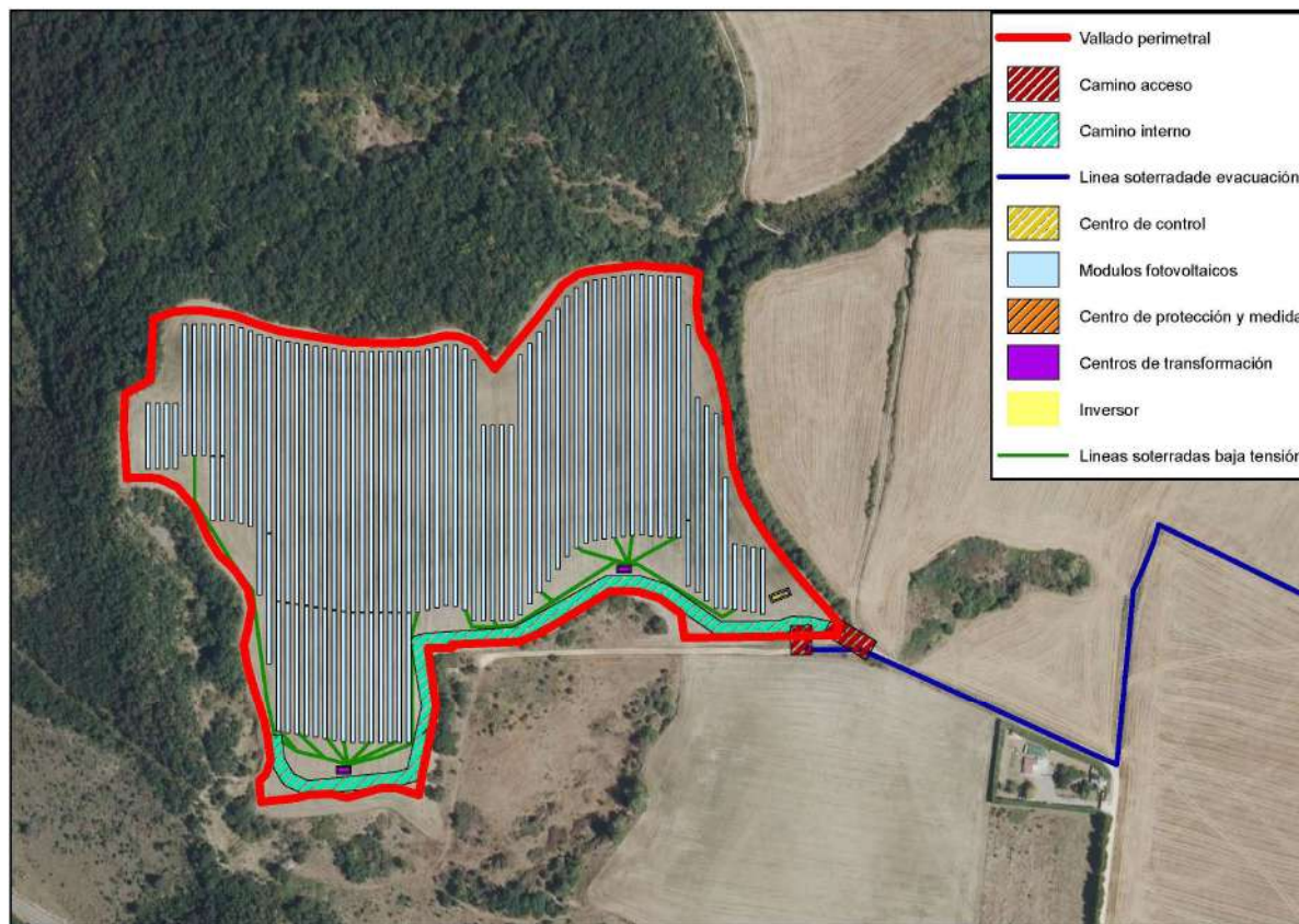
Imagen 7. Detalle de la implantación de la PSFV sobre ortofoto
