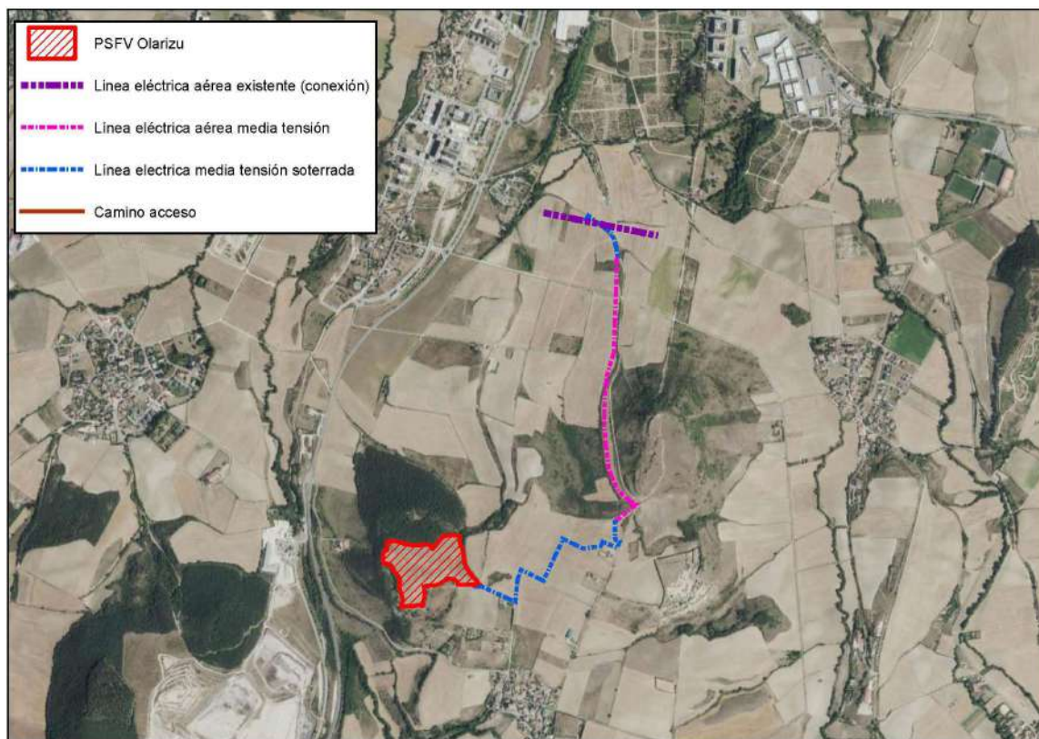
Imagen 5. Implantación del proyecto sobre ortofoto
