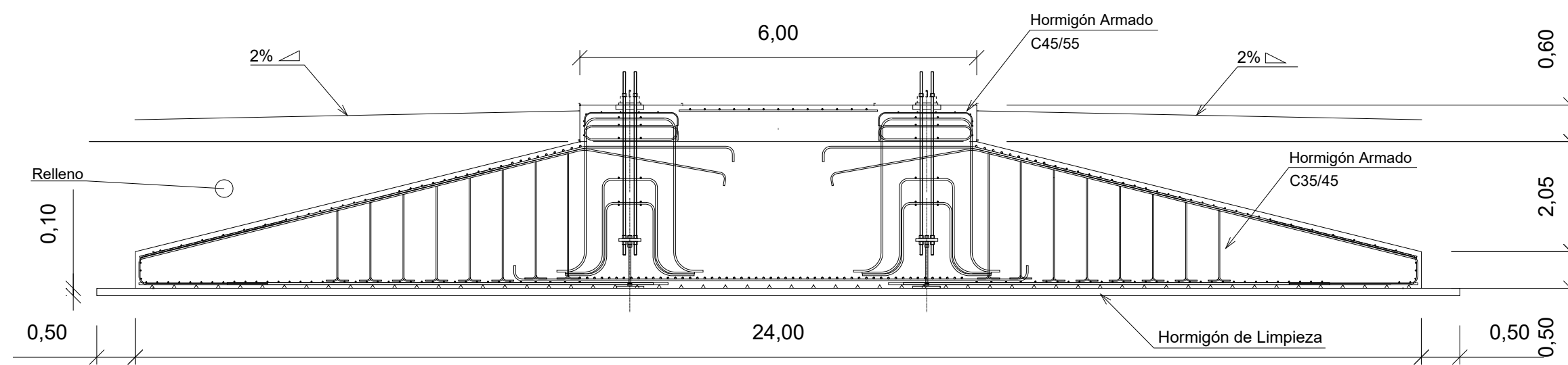
SECCION AA
