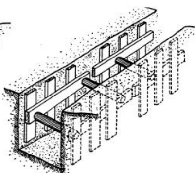
ENTIBACIÓN SEMICUAJADA
