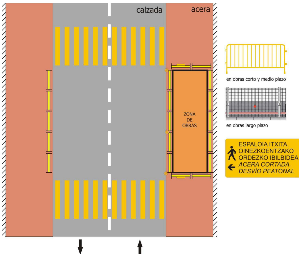
Ficha 6.2: Corte de acera y desvío por la otra acera
