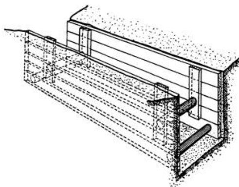
ENTIBACIÓN CUAJADA
