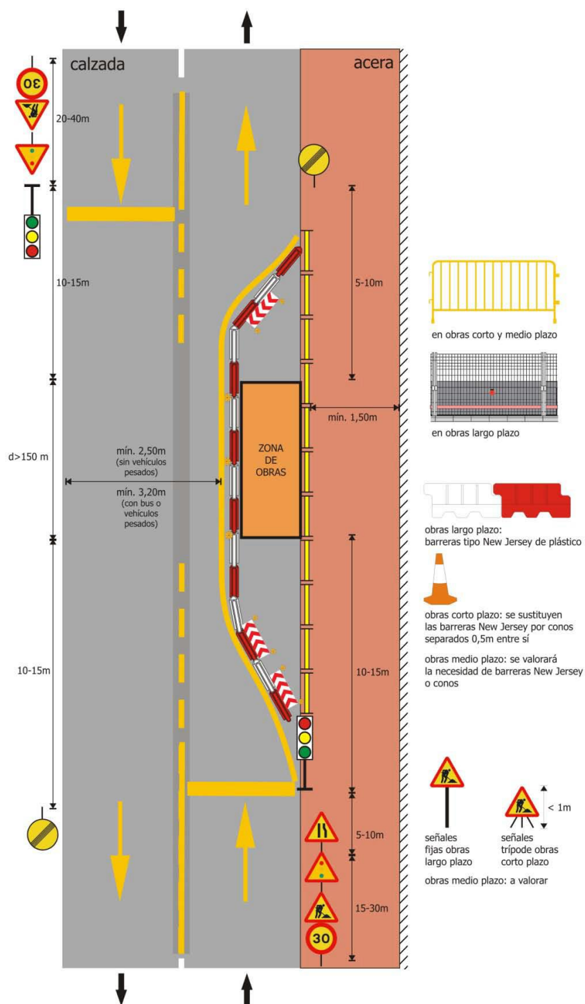
Ficha 4.1.3: En vía de doble sentido de circulación (con semáforos)
