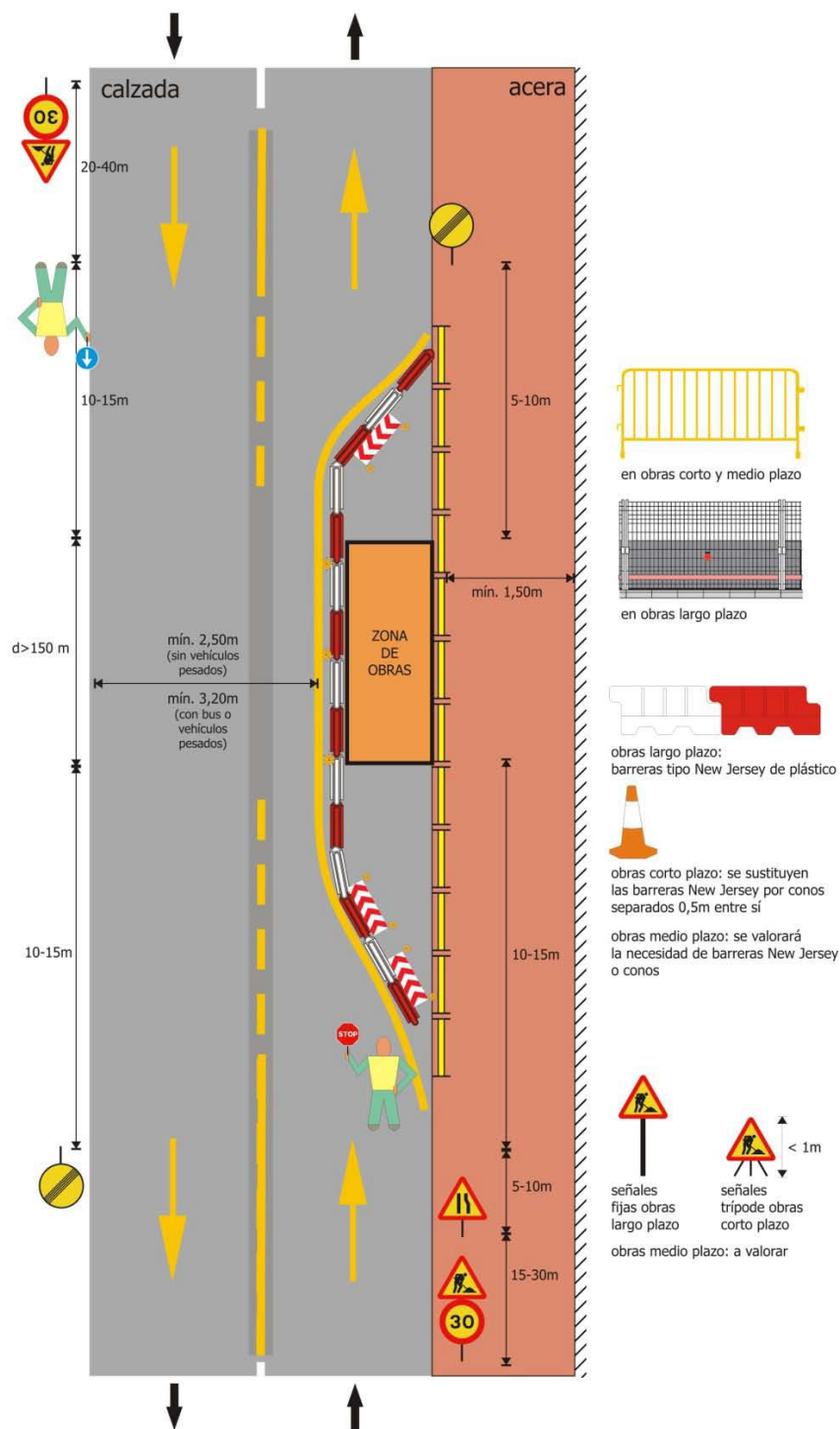
Ficha 4.1.2: En vía de doble sentido de circulación (con señalistas)
