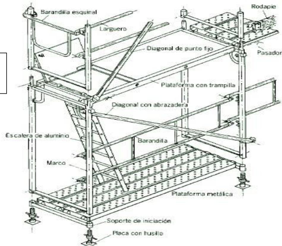
Partes de un andamio fijo prefabricado sistema modular
