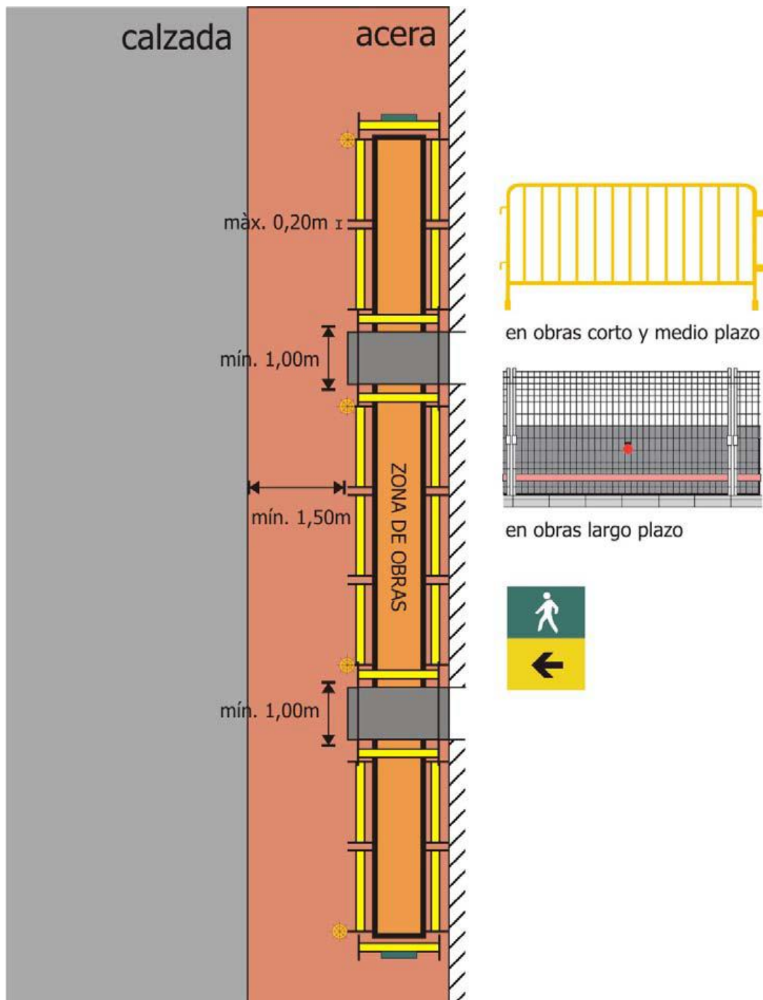
Ficha 6.1: Estrechamiento de acera
