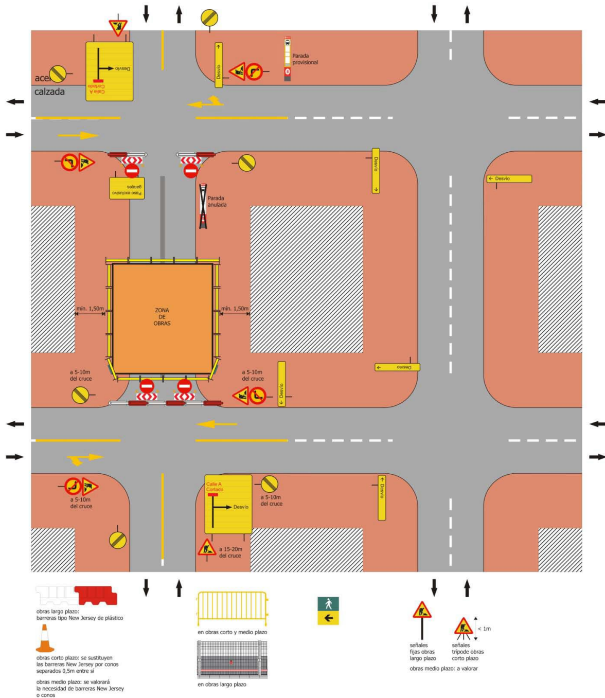
Ficha 5.1: Corte de calle y desvíos
