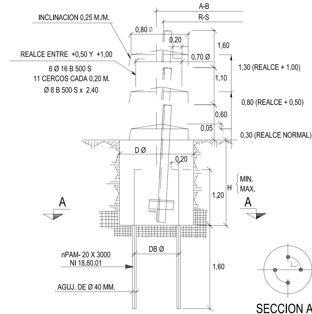
SECCION A-A
