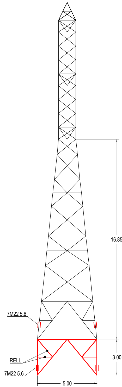
VISTA LATERAL
