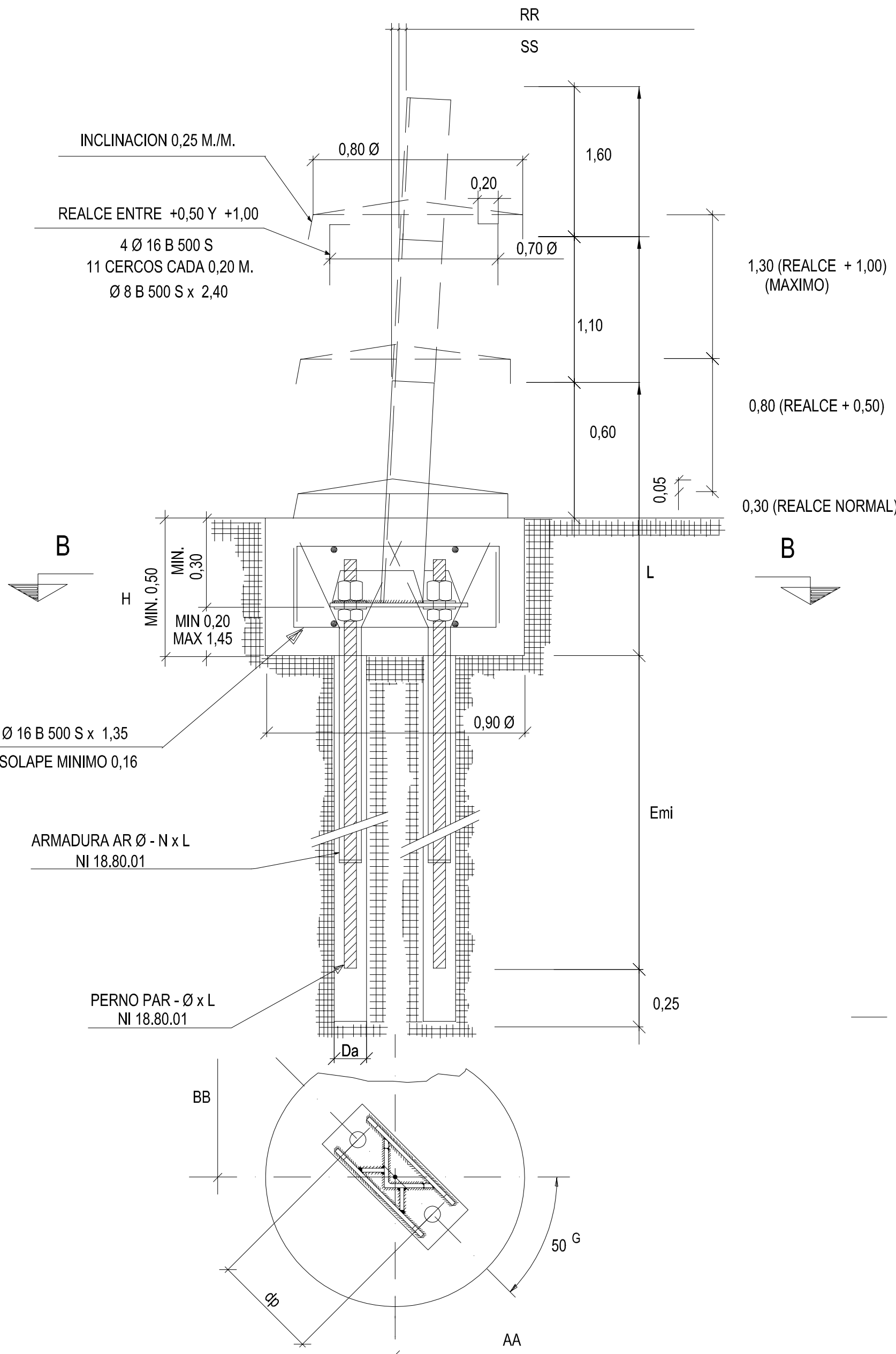
SECCION B-B
