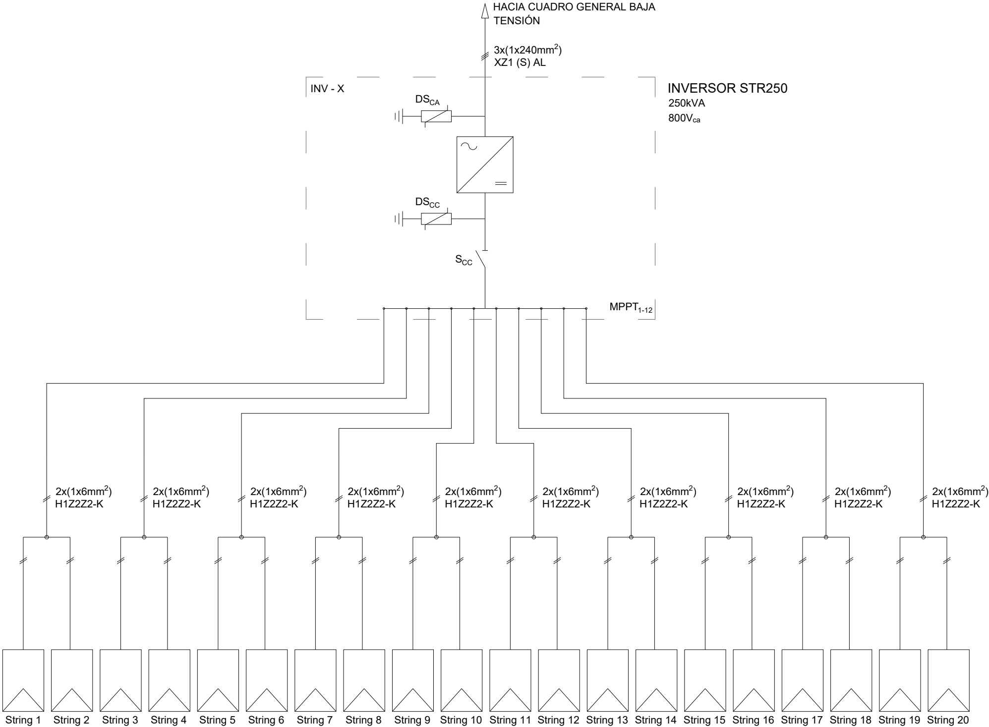
INVERSOR STR250
