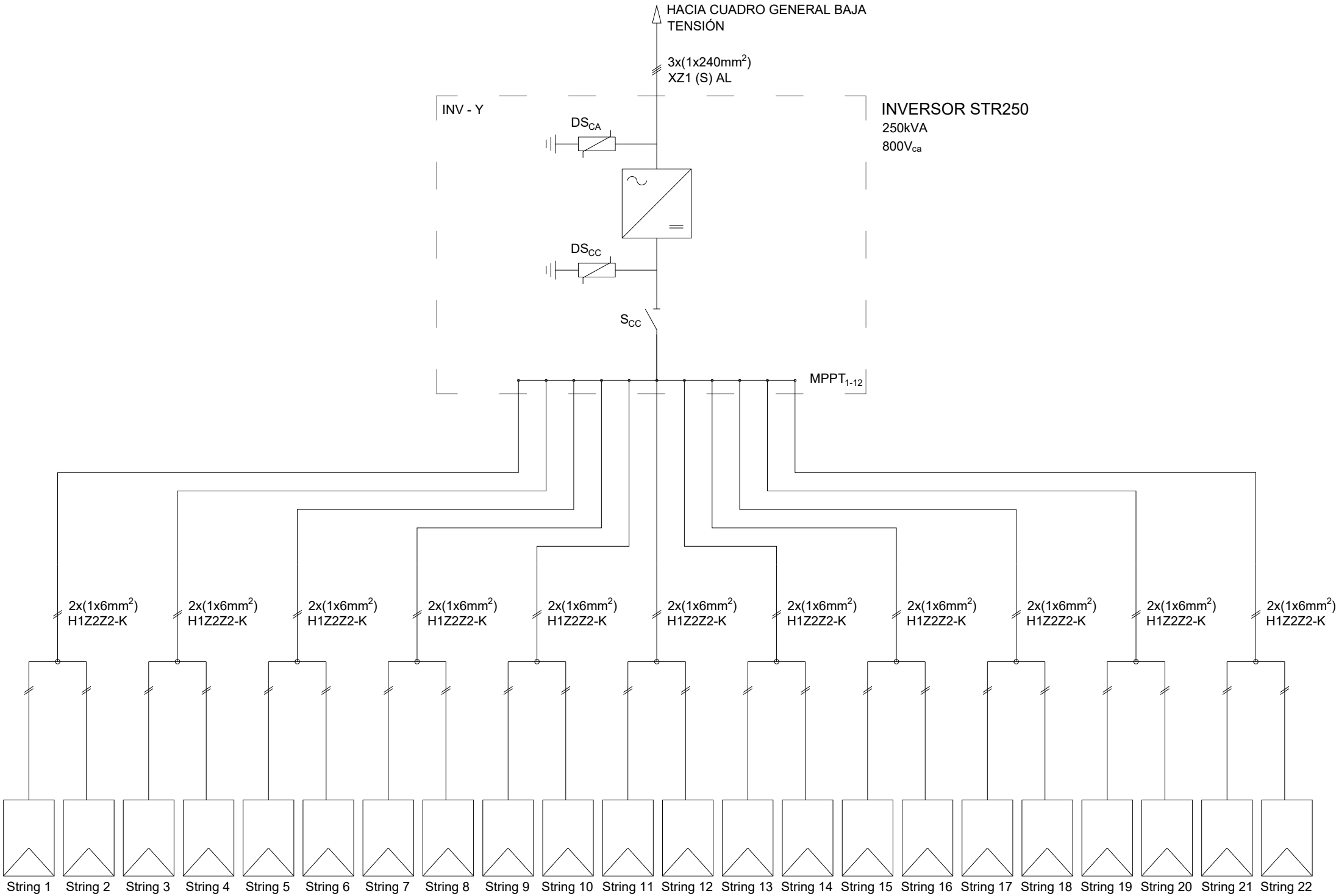
INVERSOR STR250
