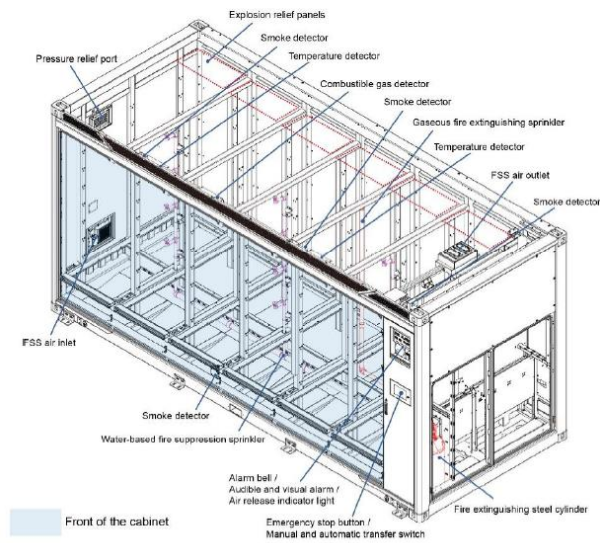
Ilustración. Disposición general del sistema antiincendios
