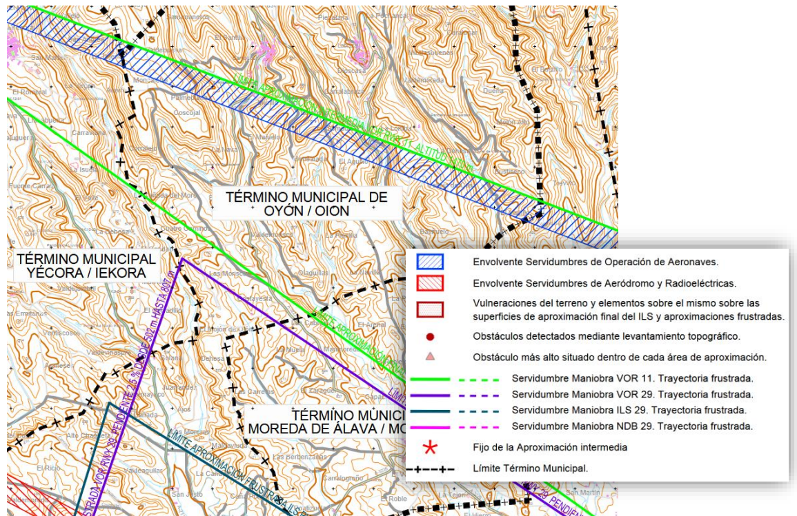
Ilustración. Situación Aeropuerto Burgos
