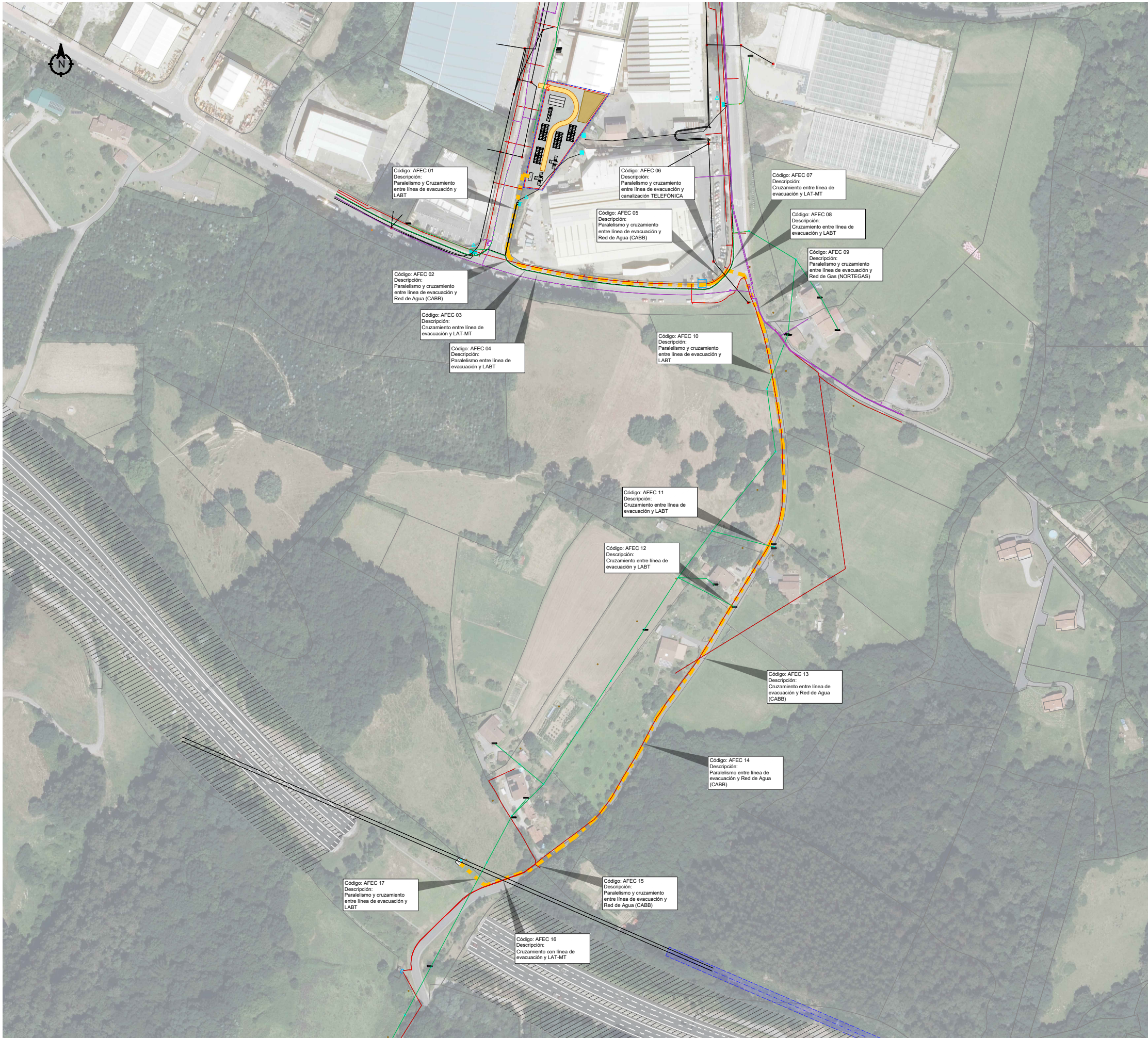
PLANTA GENERAL - RBDA ESCALA 1/1.500
